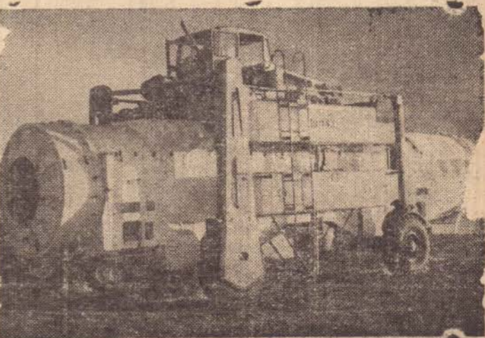
O equipamento para movimentar foguetes é quase tão complexo quanto os próprios foguetes, como o leitor pode ver por este transportador do projétil "Polaris". Este foguete de duas fases e de combustível sólido é usado por submarinos; tem um alcance de 1900 a 2400 quilômetros. Um total de nove submarinos capazes de lançar o "POLARIS" já estão em operações ou em fase de construção nos Estados Unidos.
