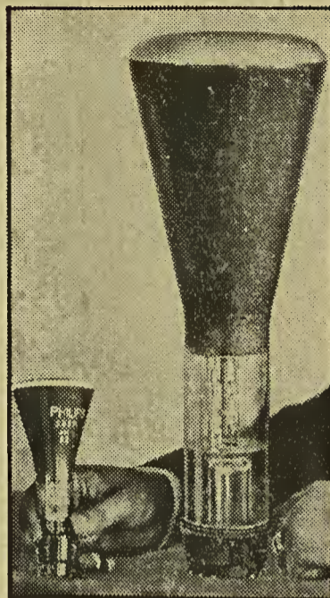
Die Kleinste und ihr grosser Bruder. — Kathodenstrahlröhren, die in Messgeräten (Oszillographen) vielfach Verwendung finden und auch von den Fernseh-Empfängern her bekannt sind, werden auf der Funkausstellung in besonders kleiner, aber für praktische Verwendung bestimmter Ausführung gezeigt.
