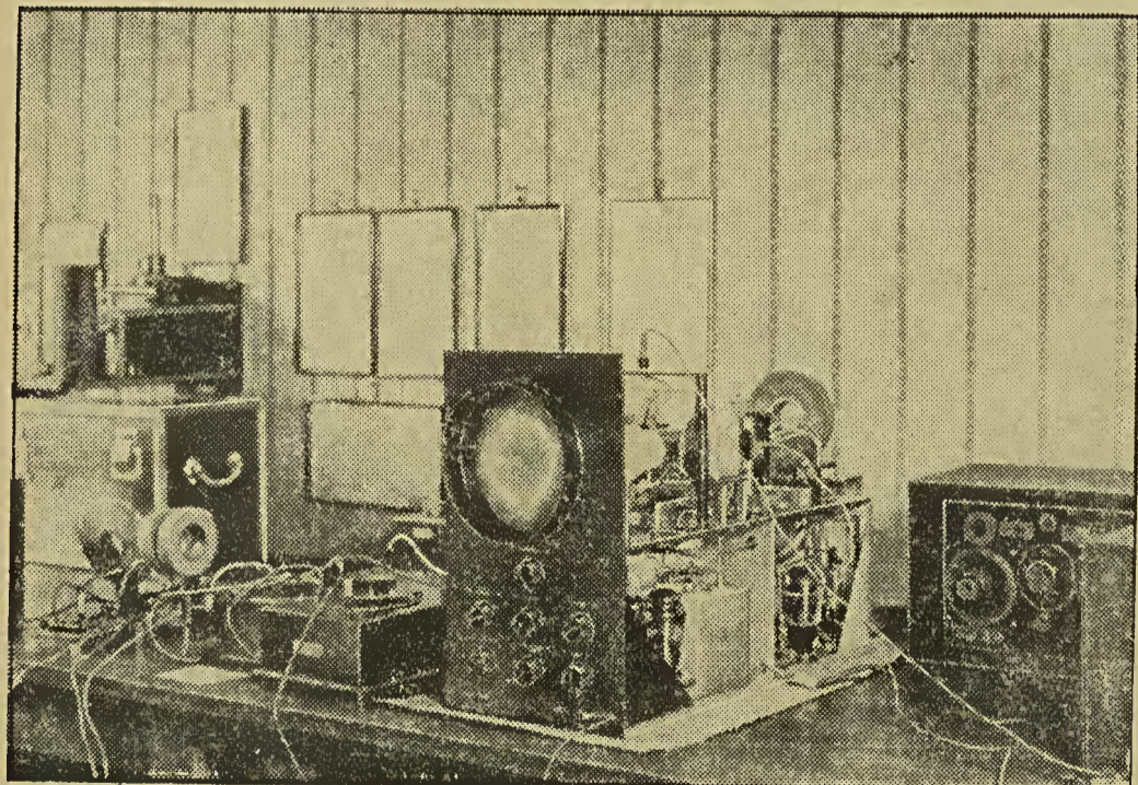
Eine Uhr, die eine zehnmillionstel Sekunde anzeigt! — Auf der Rundfunkausstellung wird in der Fernsehhalle zum erstenmal die Elektronenstrahluhr Manfred v. Ardenne gezeigt. Diese Uhr erlaubt Messung von Zeiten, die kleiner sind als eine zehnmillionstel Sekunde: Ein Elektronenstoß läuft in einer Kreisbahn über das „Sifferblatt“ im Laufe einer hunderttausendstel Sekunde. Dieses Instrument bedeutet eine Umwälzung auf dem Gebiet der Messung kleinster Zeiten.
