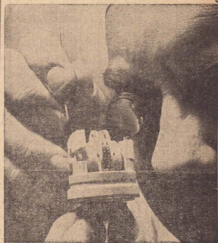
GIROSCÓPIO DE MOVIMENTO LENTO — Um cientista ajusta cuidadosamente um giroscópio de 226,8 gramas destinado a detectar a medir o movimento imperceptível do ponteiro de horas de um relógio. Os engenheiros da Companhia Mineapolis Honeywell, que aperfeiçoaram o giroscópio para orientação de foguete e naves do espaço, dizem que sua extrema precisão é essencial para as missões do espaço. Esta precisão se consegue por meio da utilização de um material de cerâmica da resistência da safira e fazendo flutuar as partes móveis sobre um tênue filme de gás hélio.
