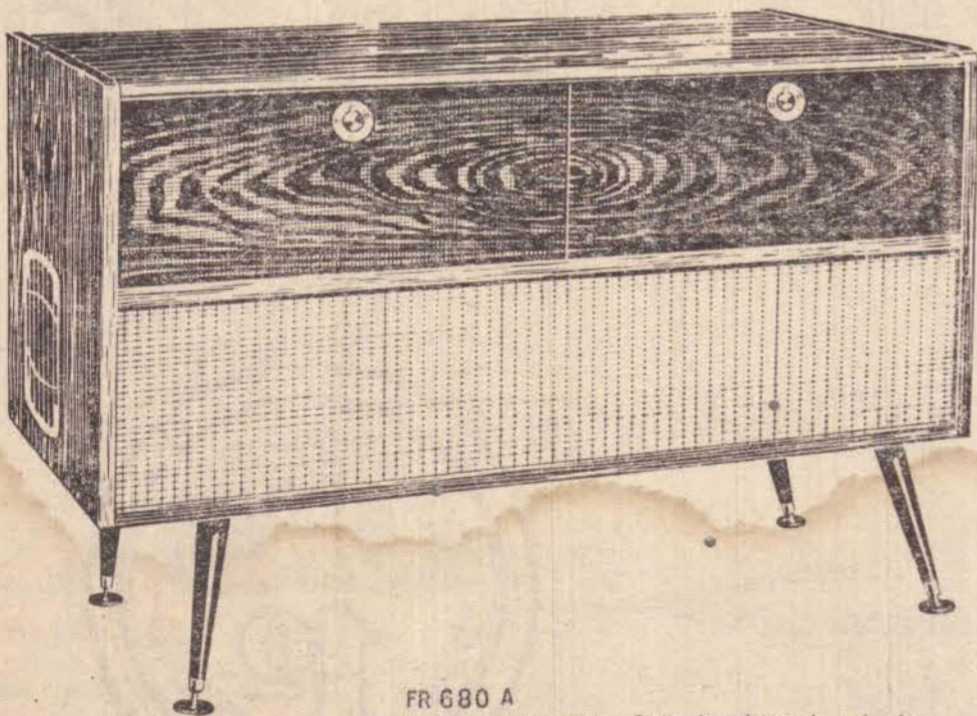
FR 680 A Radiofone estereofônico. Rádio de 6 faixas de ondas (uma de FM). Cambiador automático de 4 velocidades. 12 válvulas e 1 diodo de germânio. Extraordinária sensibilidade.
