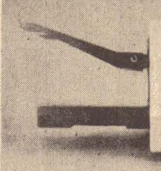
Cada cassette pode ser carregado com um tipo diferente de papel, facilitando a troca rápida de um tamanho para outro.
