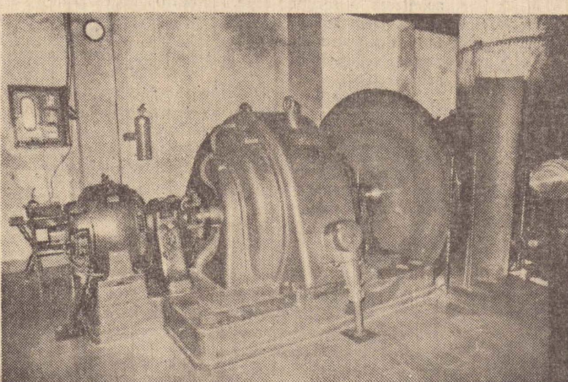
A foto nos mostra o gerador da Usina Laranja Doce. Essa hidrelétrica foi inaugurada em 1930, quando a Caiuá iniciou, propriamente, o fornecimento de energia elétrica em maior área regional.
