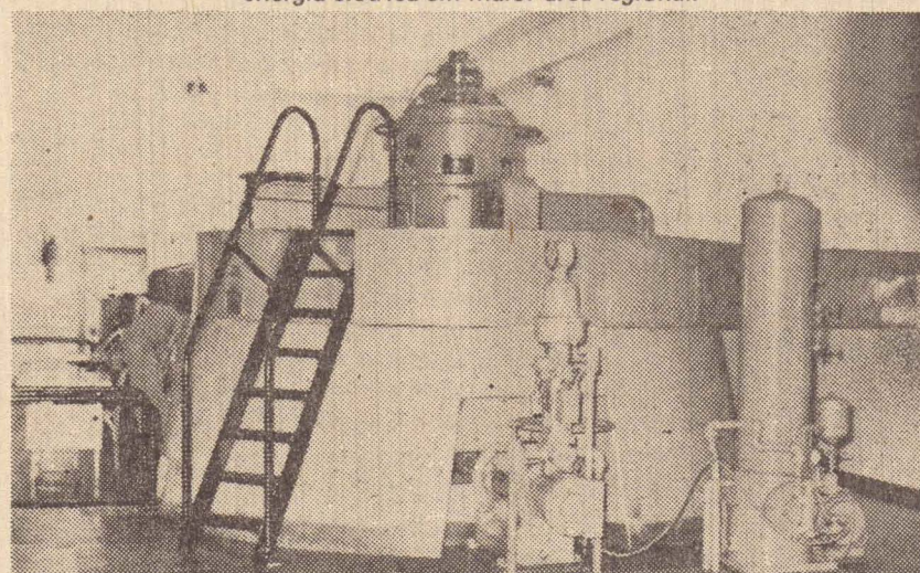
Inaugurada em 1940 a Usina Quatiara, represamento do rio do Peixe, é uma das grandes geradoras da Caiuá. Ai está um dos conjuntos de turbina e gerador daquele completo hidrelétrico.
