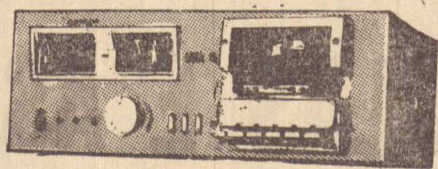
Cassete - deck frontal metal-compatível e com acesso direto. Ajuste para fita de metal - Front-Load - Acesso direto ao compartimento de fita (Direct-Access) - Sistema Dolby NR - parada automática em qualquer modo de operação - Cabeças Metarpen - Motor DC com governador eletrônico - Controlador de fita.
