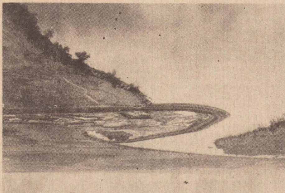
A execução da ensecadeira representa uma das fases mais importantes da futura Hidrelétrica de Capivara, que a partir de 1.973 receberá equipamentos técnicos russos.
