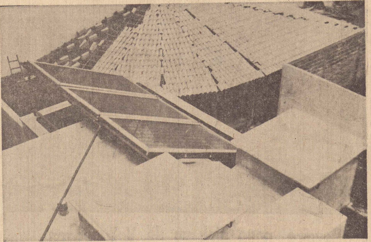
No telhado da residência, a placa que absorvem a energia do sol para aquecer a água que vai para um reservatório térmico ficando a disposição para o uso doméstico
