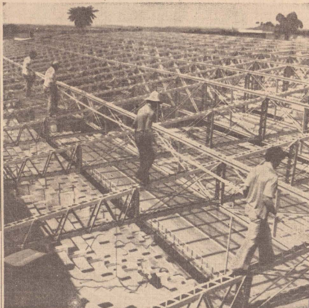
Pessoal especializado da Prefeitura Municipal de Presidente Prudente, está executando completa reforma na estrutura metálica da cobertura do Ginásio Municipal de Esportes, com vistas às próximas promoções de cunho social-esportivo. O trabalho exigiu intensos esforços por vários dias, mas já está quase concluído.
