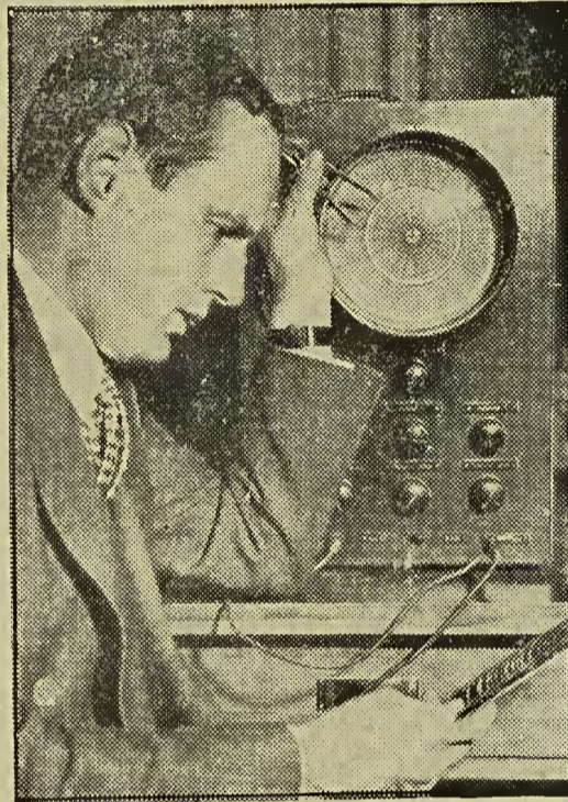
Der genaueste Zeitmesser. — Die Elektronenuhr stellt eines der genauesten Zeitmessgeräte der Welt dar, die die moderne Technik kennt. Eine Zeitdifferenz von einer sechzigmillionstel Sekunde, das ist die Zeit, die ein Lichtstrahl braucht, um fünf Meter zurückzulegen, wird von diesem Gerät gemessen. Vor dem Gerät sein Erfinder Manfred v. Ardenne.
