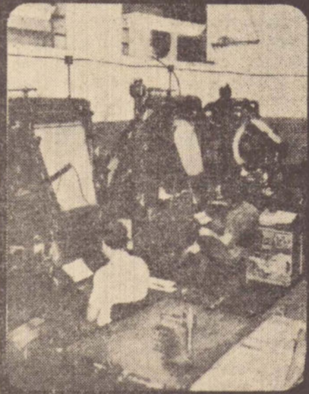
Composição a Quente - Linotypia
