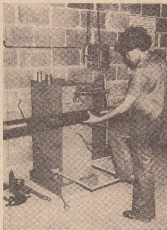
A fixação dos contra- pesos, proporciona equilíbrio dinâmico com precisão absoluta.
