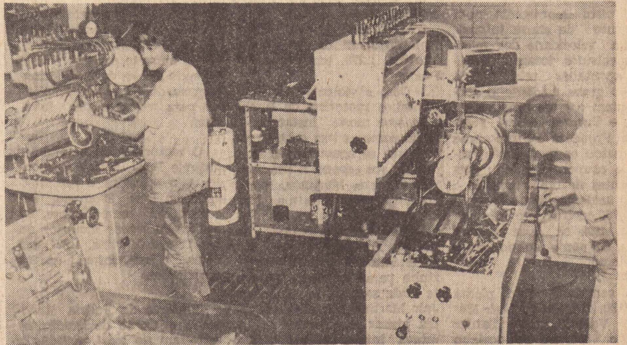
Esta foto nos dá uma amostragem do funcionamento da bancada de testes para regulagem de bombas injetoras. Em primeiro plano, o conjunto de máquinas, de fabricação da própria BOSCH, no Brasil, e que põe em evidência a "Boa Estrela Eletrodiesel, Ltda." pois é a única existente em nossa região. Essas máquinas operam com muito mais eficácia e rapidez.
