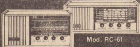
Mod. RC-61 Rádio de mesa e cabeceira com 6 faixas de onda. Pilha e Luz. 110/220 volts. Gabinete em madeira de lei. Som em HI-FI.
