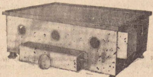
CHAPA PARA FRITURAS Aparato em aço INOX para preparar baurus, bifes, ovos, frituras em geral. Comp: 0,40 — Larg: 0,30 e alt: 0,20 cms.
