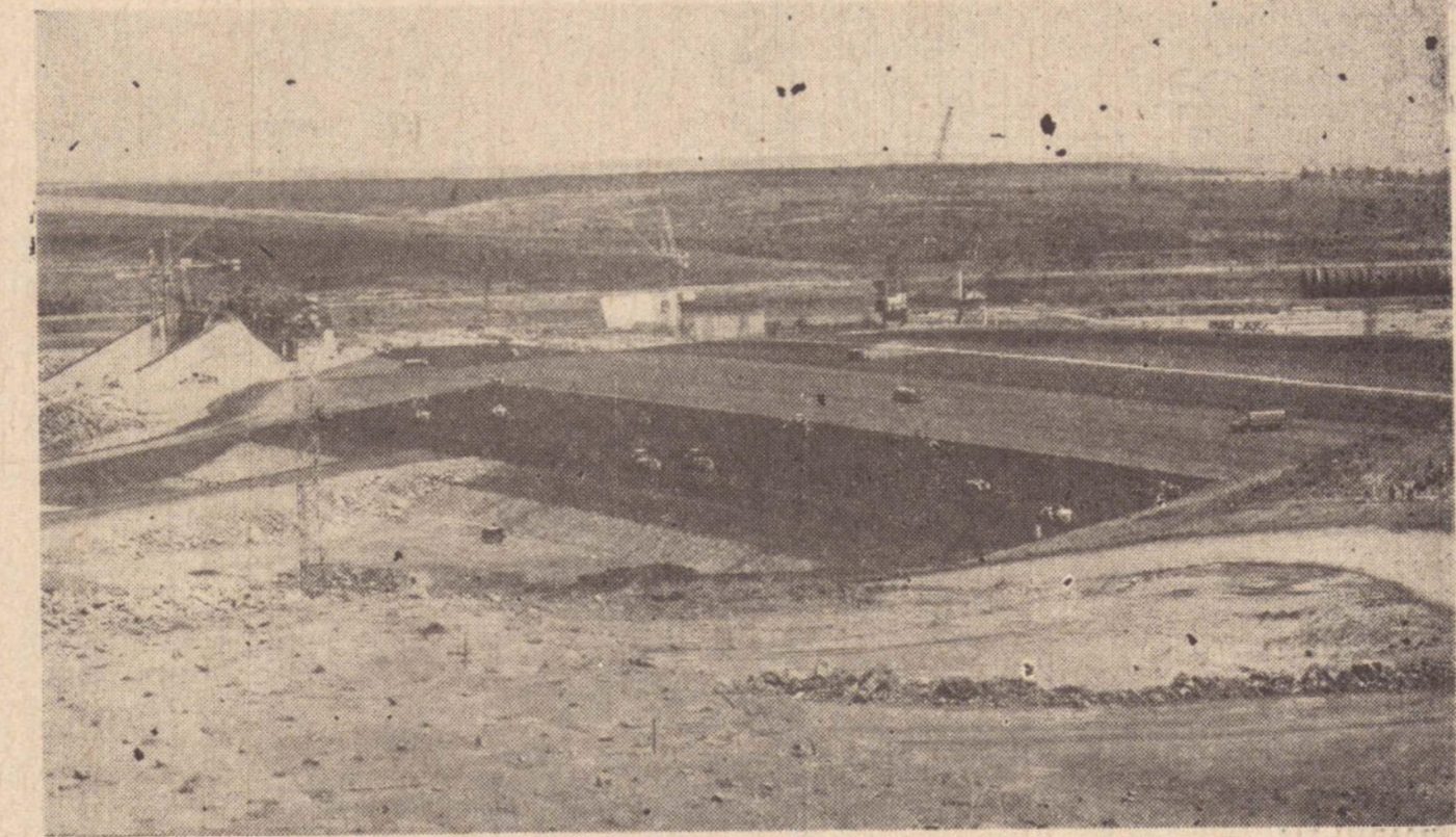
As máquinas trabalham na compactação de argila. A direita será construída a barragem de 1,5 km.
