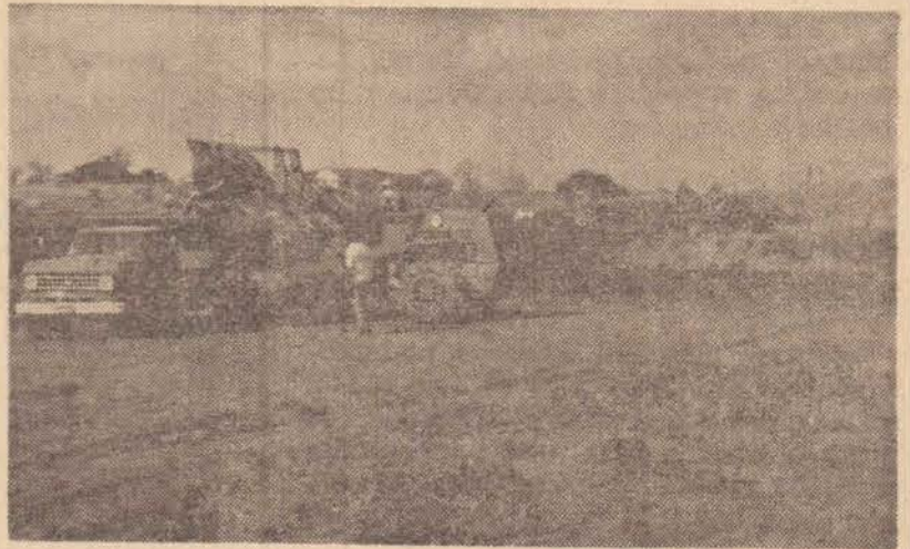
Regularização do fundo da 2.ª lagoa de recuperação de qualidade (ERQ) em Lucélia.
