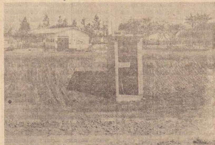
A nova tomada d'água que demandou 20.000 m 3 de escavações para preparo das fundações, 48 m 3 de concreto, 226 m 2 de forma e 3.300 kg de aço.
