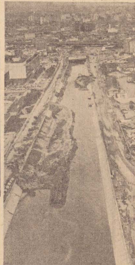
Canalização do Rio Tamanduateí — DAEE — Vista geral da obra e concretagem dos taludes das margens.
