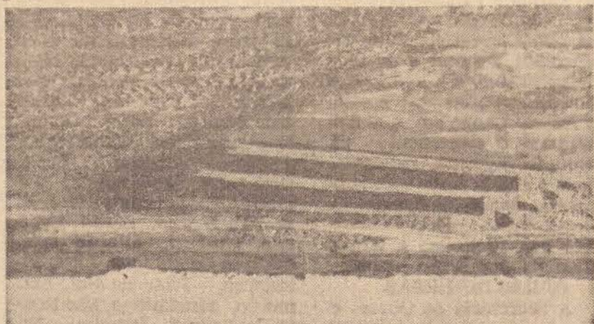
Aqui, uma visão geral do vertedouro de emergência que demandou um volume de 606 m 3 de gabiões dispostos em escadas para dissipar energia e 614 m 3 de enrocamento para proteger o canal.
