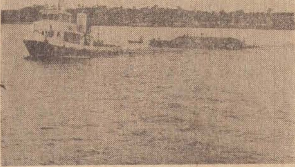
A CESP — Companhia Energética de São Paulo lançou às águas do rio Paraná a maior comporta flutuante do mundo. O "stop-log", como é chamado, tem uso na vedação de vertedouros para os trabalhos de manutenção.
