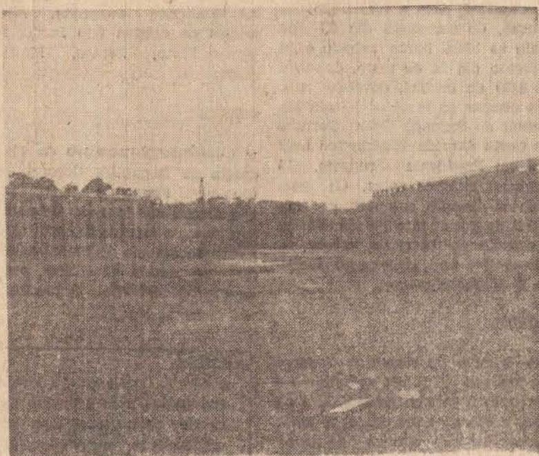
Vista parcial da obra do depósito de Cotia, na qual aparecem duas linhas de colunas com as vigas calhas e os locais de moldagem dos pré-moldados.
