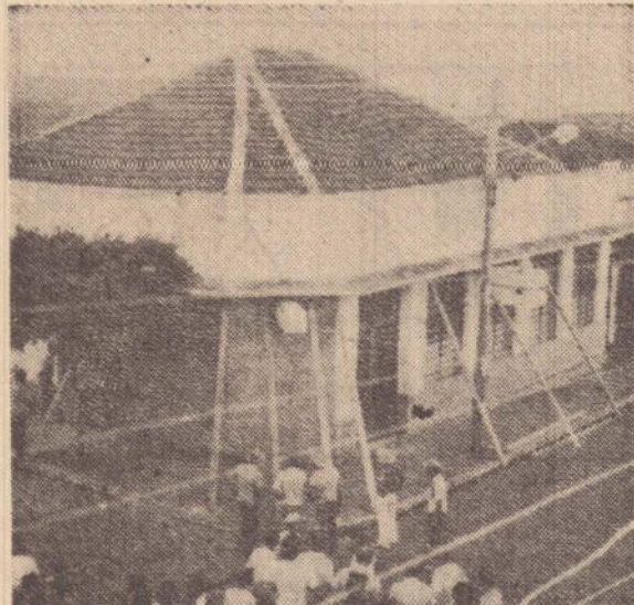
Devido a fendas produzidas na marquise do edifício, ela passou a ser escorada por eucaliptos.
