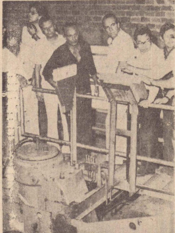
O interior da usina pioneira de alcool anidro, no Pontal do Estado, o Ministro das Minas e Energia, o governador do Estado, o eng. Lamartine Navarro Jr. e convidados.
