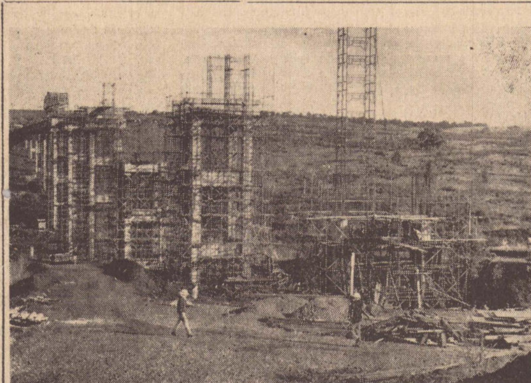
CESP constroe ponte para dar passagem a geradores da usina
