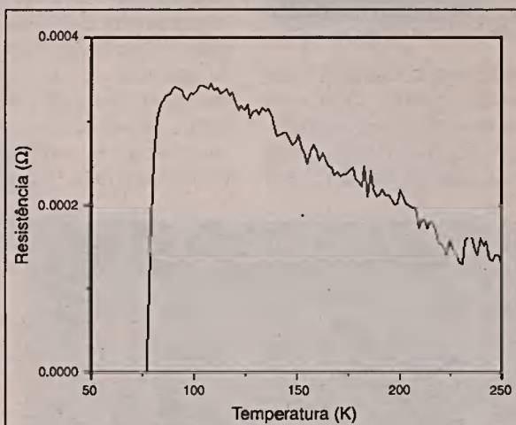
Gráfico da resistência em função da temperatura. Pode-se observar que em torno de 80 K ocorre uma queda muito acentuada da resistência, que tende a zero. Essa queda acentuada ou abrupta é conhecida como transição supercondutora, ou seja, o material passa do estado condutor (semelhante ao dos metais) para o estado supercondutor dos materiais cerâmicos.
