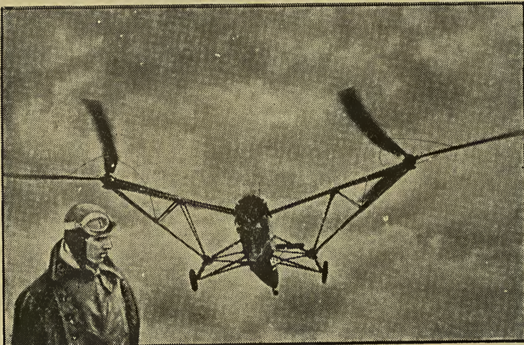
Großerfolge der deutschen Luftfahrt — Deutscher Hubschrauber bricht sämtliche Rekorde. — Mit einer von Prof. Heinrich Focke erbauten Hubschraubenkonstruktion brach der Flugzeugführer Rohls (links) sämtliche für diese Flugzeuggattung geführten internationalen Rekorde. Er erreichte 2500 Meter Höhe, flog 1 Stunde 20 Minuten 49 Sekunden lang, erreichte eine Geschwindigkeit von 122,5 Kilometerstunden, legte eine Entfernung in gerader Linie von 16,4 Kilometer zurück und brachte es einschließlich Rückkehr auf einen Flug von 80,6 Kilometer. Damit ist mit einem Hubschrauber zum erstenmal ein größerer Ueberlandflug durchgeführt worden.
