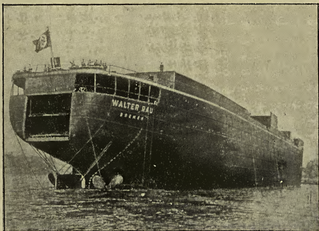
Das erste deutsche Walfang-Mutterschiff lief vom Stapel. — Auf der Deutschen Werft in Sanktwarder lief das erste deutsche Walfang-Mutterschiff vom Stapel. Der Neubau, der eine Größe von 22 000 Tonnen hat, ist 175 m lang. Er wurde von Frau. Rau auf den Namen „Walter Rau“ getauft. Der Reichsstatthalter von Bremen und Oldenburg, Gauleiter Röber, hielt die Taufrede. — Das neue Walfang-Mutterschiff in seinem Element. Deutlich sieht man am Heck die riesige Öffnung, durch die die erlegten Wale an Bord gezogen werden.
