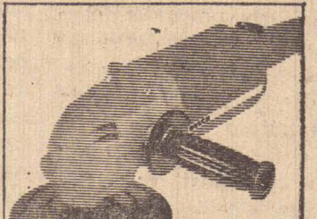
Lixeira Angular. • 1600 Watts. • Rotação: 5000 rpm. • Disco de lixa de 7" Ø. • Peso: 4,8 Kg. • Nº tipo: 1323.
