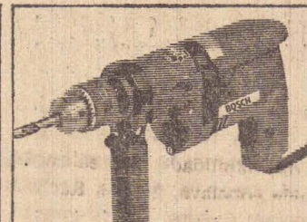
Furadeira - 2 velocidades. • 400 Watts. • Rotações: 420/1000 rpm. • Capacidade: 13/8 mm Ø em aço. • Peso: 1,95 Kg. • Nº tipo: 1111.
