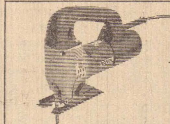
Serra Tico-Tico • 320 Watts. • Capacidade de corte: 60 mm em madeira, 30 mm em material sintético, 20 mm em metal não ferroso, 6 mm em aço doce. • golpes: 3000 gpm. • Peso: 2,6 Kg. • Nº tipo: 1577.
