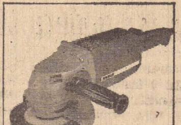
Esmerilhadeira • 2200 Watts. • Rotação: 8500 rpm. • Capacidade para disco de desbaste ou corte: 7" Ø. • Peso: 5,7 Kg. • Nº tipo: 1331.
