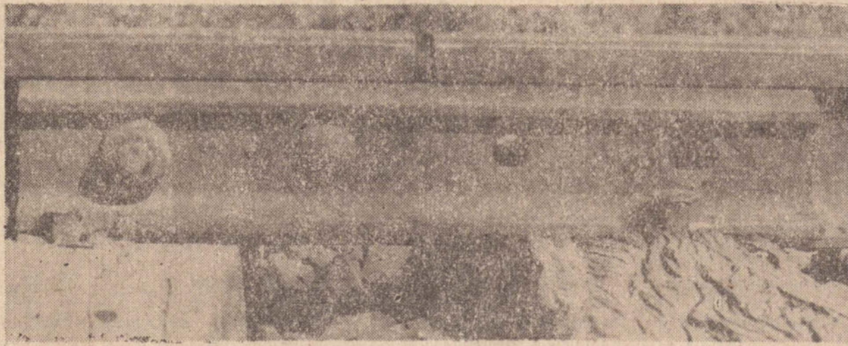
Com se vê na fotografia, foram retirados dois parafusos dos 4 que prendem uma tala na junção dos trilhos. Um dos parafusos foi afixado com auxílio de maleta no vão entre os dois trilhos.
