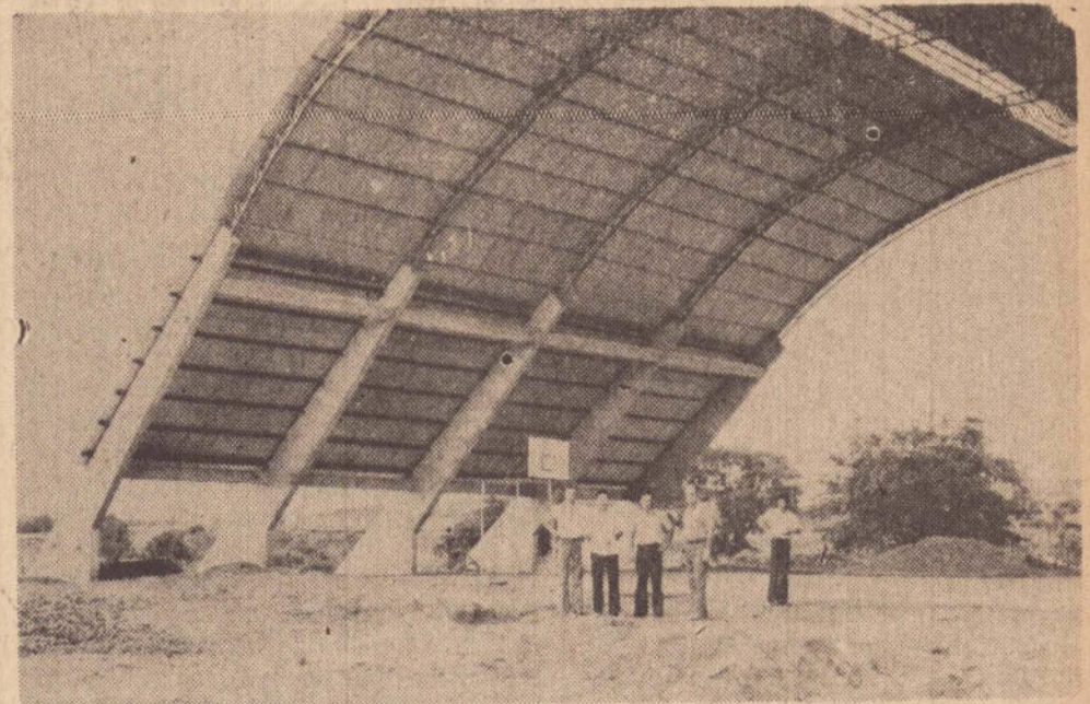
De linhas arquitetônicas e cobertura em alumínio, o Ginásio de Esportes de Santo Anastácio vai sendo construído.
