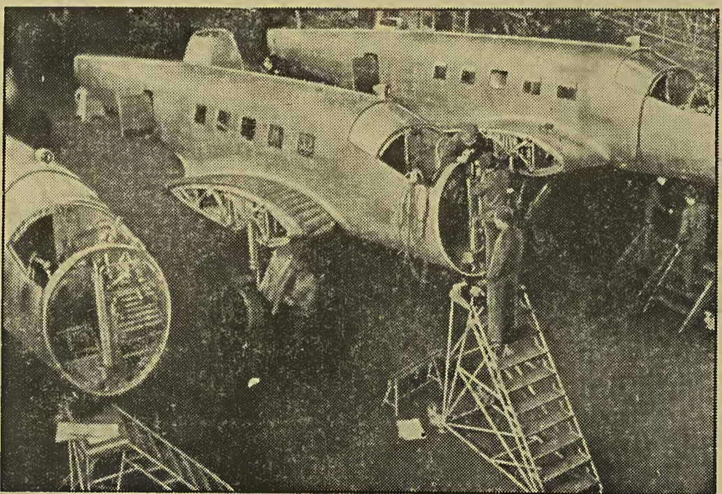
Die „Ju 86“ — das schnellste Verkehrsflugzeug im Bau. — Die südafrikanische Luftverkehrsgesellschaft hat bei den Junkerwerken drei Flugzeuge vom Typ „Ju 86“ in Auftrag gegeben, die wir hier im Bau sehen. Auf besonderen Wunsch der afrikanischen Gesellschaft werden die Maschinen mit Rolls-Royce-Motoren ausgerüstet. Damit werden sie eine Maximalgeschwindigkeit von 585 Kilometern erhalten und so die schnellsten im Luftverkehr stehenden Flugzeuge der Welt sein.
