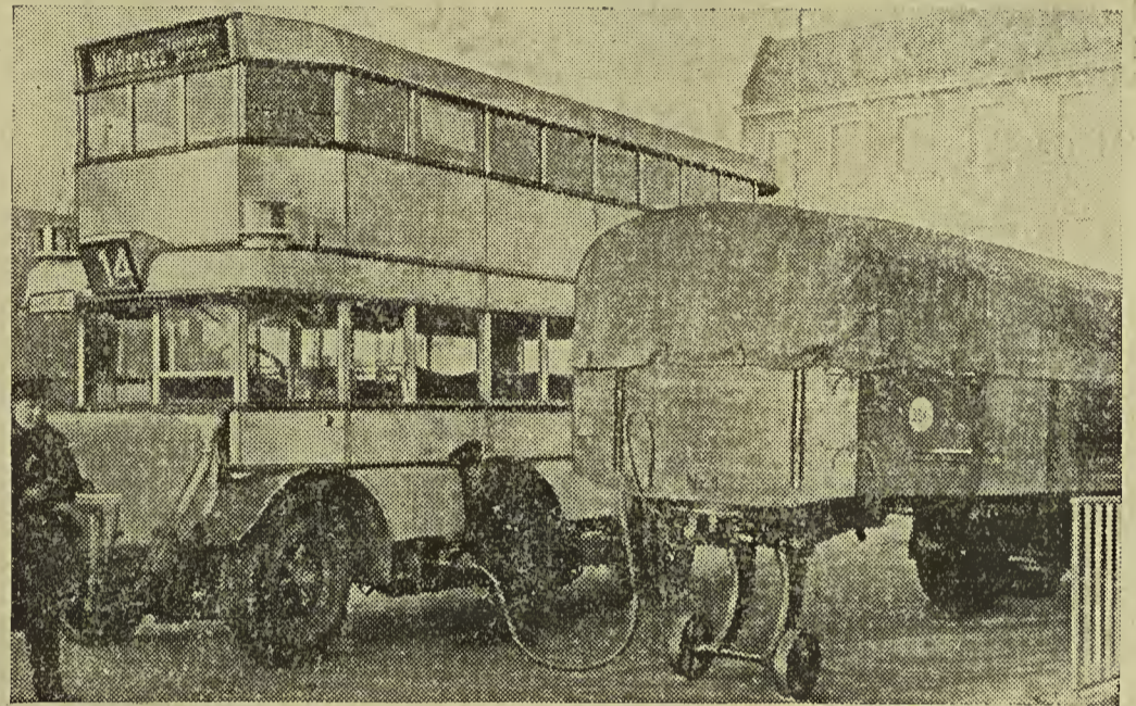
Die erste rollende Gas-Tankstelle wurde jetzt zur Versorgung der mit Stadtgas angetriebenen Omnibusse der Berliner Verkehrsgesellschaft in Betrieb genommen. Damit ist ein neuer Schritt getan, Verkehrsmittel von ausländischen Treibstoffen unabhängig zu machen.
