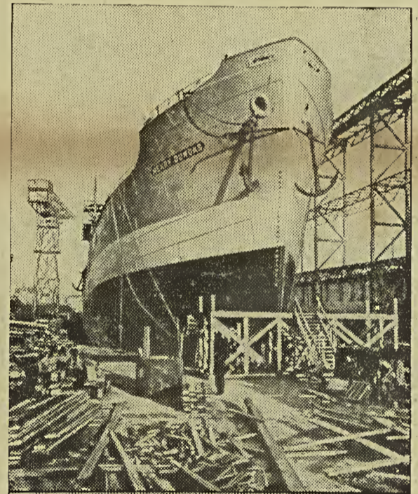
Ein Deutsches Tankschiff für einen amerikanischen Oelkonzern. Auf der Kieler Germania-Werft lief das Motortankschiff „Henry Dundas“ vom Stapel, das für die Standard Vacuum Oil Company, Neuyork, bestimmt ist und eine Grösse von fünfzehntausend Tonnen besitzt.
