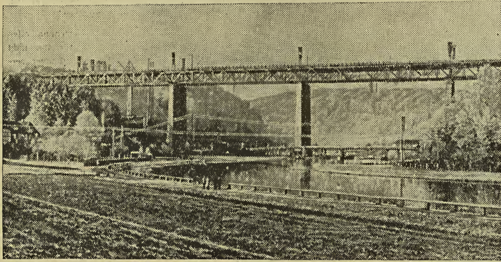
Eine neue gewaltige Brücke der Reichsautobahn. — Ein überragendes Bauwerk im Zuge der Herstellung der Strassen des Führers ist nunmehr mit der grossen Autobrücke, die in der Nähe von Hannoversch-Münden die Werra in einer Höhe von 60,80 Meter überquert, fertiggestellt. Die Brücke ist 416 Meter lang. Die Breite zwischen den Geländern beträgt 21,50 Meter. Die zwei Fahrbahnen von je 7,50 Meter Breite sind durch einen erhöhten Mittelstreifen von drei Meter getrennt.
