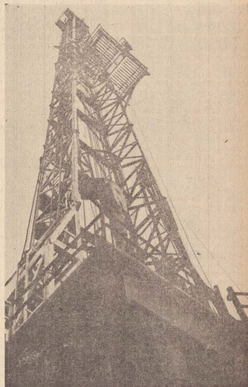
A torre do poço de Cuiabá Paulista, com 50 metros de altura, cuja sonda deverá perfurar até 6 mil metros.
