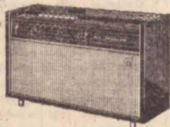
B 4 R 05 T - 4 faixas. Transistorizado. Tomada para tocas-discos. 2 antenas internas. Comando e seleção de faixas por tocas. Alimentado por 6 pilhas. Adaptável ao uso em corrente alternada.
