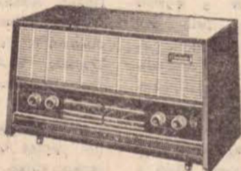
B 4 R 06 A - 5 válvulas com funções de 8. Duas antenas. 3 faixas de ondas. Tomada para tocas-discos. Possante alto-falante. Grande cobertura de frequências. Magnífica sonoridade. 110/220 Volts.
