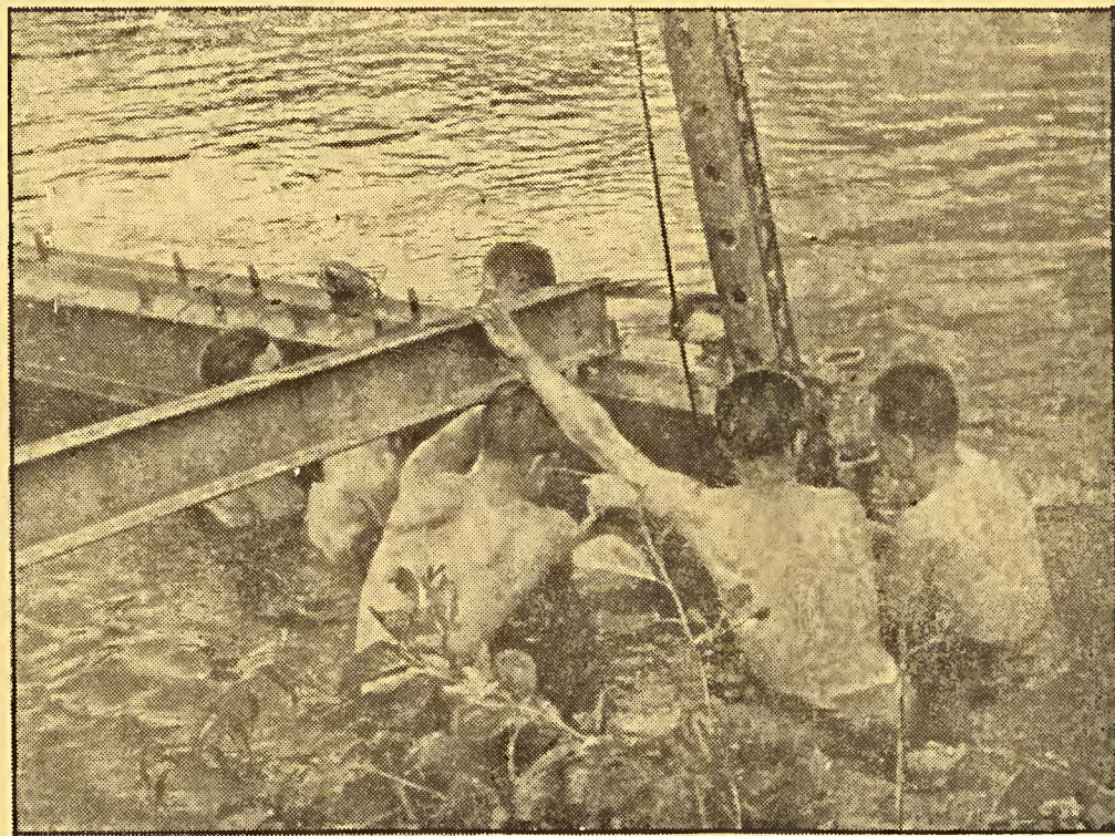
Bis zu dem Bauch im Wasser stehend. — Eine von den Polen bei ihrem Rückzug gesprengte Brücke muss in Eile ersetzt werden. Bis zu dem Bauch im Wasser stehend, arbeiten unsere Pioniere fieberhaft.
