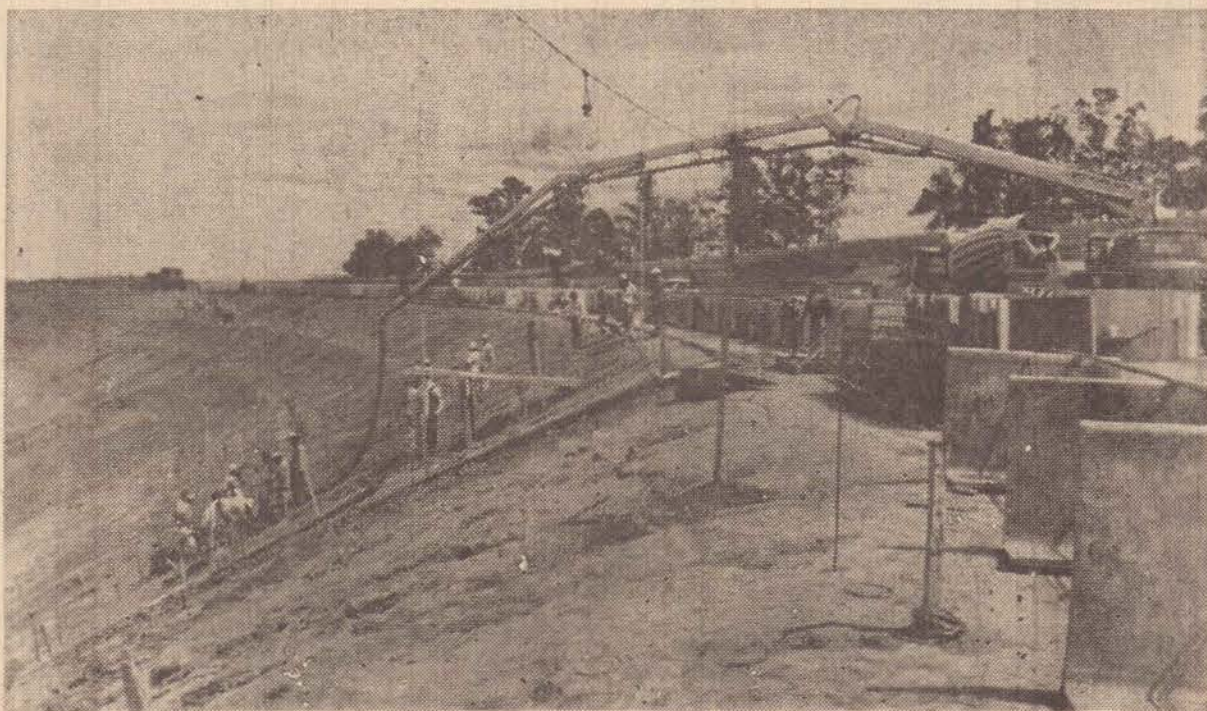
O concreto desce para as perfurações diretamente da betoneira, através de uma canalização.
