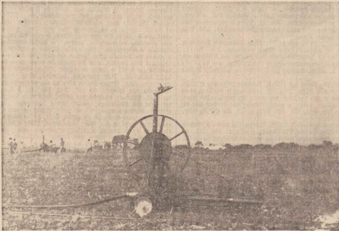
O "Chuvisco" projetado para irrigar área de até 30 hectares, da linha Perromatic.
