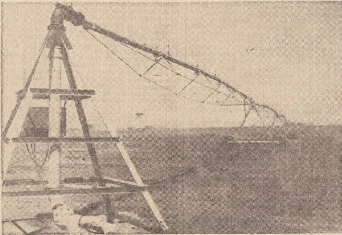
Irrigação automática por aspersão — Sistema pivot central, movimentando-se em círculo, cobre uma área de 32 alqueires
