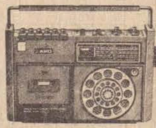
AIKO ATRP-405 - RÁDIO/GRAVADOR portátil AM/FM/SW, microfone embutido, monitor, filtro de ruídos, pausa, pilha/luz.
