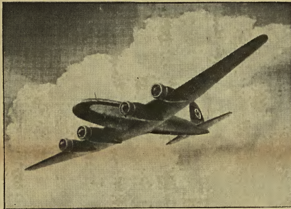
Ein neues deutsches Großflugzeug: Focke-Wulf „Condor“. — Da der ständig steigende Platzbedarf auf den internationalen Flugstrecken der Deutschen Luft Hansa es notwendig gemacht hat, neue Großflugzeuge zu schaffen, ist jetzt dem Großflugzeug „Ju 90“ ein weiteres Großflugzeug der Focke-Wulf-Flugzeugbau gefolgt. Das viermotorige Großflugzeug S. W. 200 „Condor“ ist ein Ganzmetalltieflieger, dessen ausgezeichnete aerodynamische Durchbildung eine Durchschnittsgeschwindigkeit von 345 Stundenkilometer ermöglicht. In den beiden geräumigen Kabinen der Maschine finden 26 Fluggäste Platz.
