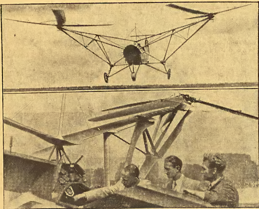
Weltrekord des Focke-Hubschraubers. — Der von Prof. Focke geschaffene Hubschrauber erlangte der deutschen Luftfahrt eine neue Weltbestleistung: Mit 230 Kilometer stellte Dipl.-Ing. Bode einen neuen internationalen Streckenrekord auf. — Unten: Prof. Focke (links) und Dipl.-Ing. Bode (Mitte) an der erfolgreichen Maschine. Oben: Der Hubschrauber.
