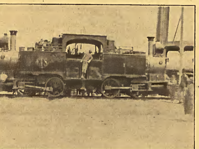
Die erste Lokomotive der Sorocabana, die für Vorwärts- und Rückwärtsfahrt zwei Dampfkessel und zwei Schornsteine benötigte
