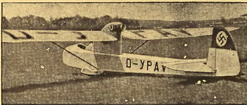
Segelflugzeug mit Motor. — Aus dem Berliner Flughafen Rangsdorf führte der bekannte Segelflieger Ludwig Hofmann die Neukonstruktion eines Segelflugzeuges mit Motor vor, die ausserordentlichen Beifall erntete. Der Zwei-Zylinder-Motor ist 800 Kubikzentimeter stark und verleiht der Maschine bei 8 Liter Verbrauch auf 100 Kilometer eine erstaunlich hohe Geschwindigkeit.
