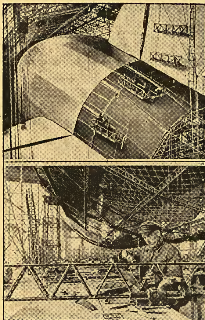
„LZ 130“ vor der Vollendung. — Seit anderthalb Jahren ist in der riesigen Montagehalle des Luftschiffbaues in Friedrichshafen der neue deutsche Luftriese „LZ“ 130 im Bau, der nach dem vorläufigen Fahrtenprogramm der deutschen Zeppelinreederei noch in diesem Jahre mehrere Reisen von Frankfurt nach New York und zurück antreten wird. Oben: Arbeiten am Heck des Luftschiffkörpers. Unten: Ein Blick in die riesige Werkhalle. Im Vordergrund: Ein Arbeiter beim Vernieten eines Aluminiumträgers.
