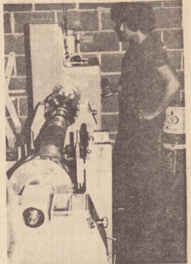
Balanceamento do Cardan, depois de alinhamento
