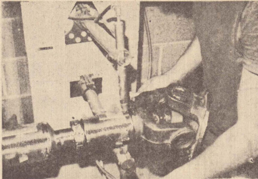
Fixação de contra — pesos, depois de balanceado o Cardan
