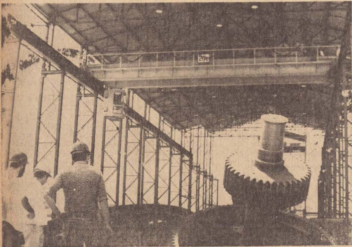
Ainda aguardando montagem, aparece neste ângulo fotografico as engrenagens redutoras para o acionamento dos termos de moega. No plano superior, é vista a ponte rolante, que funciona a 12 metros de altura e com capacidade para 20 toneladas.
