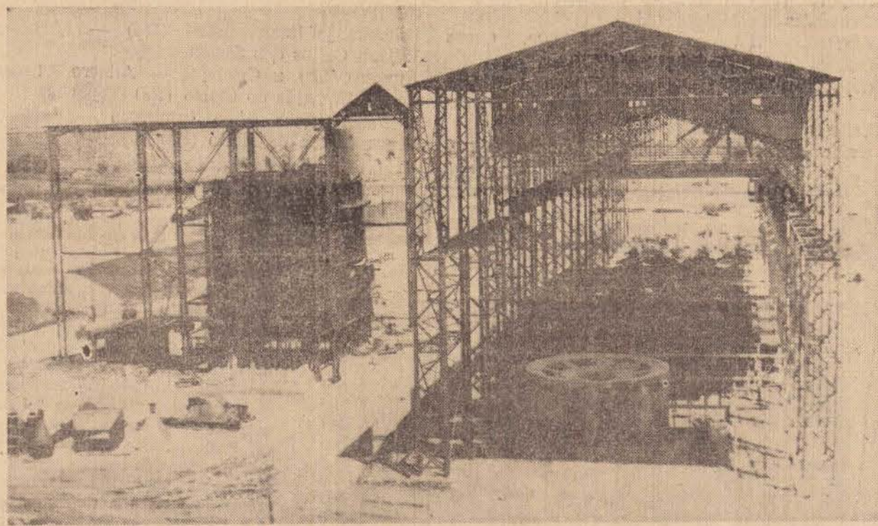
Ao centro, o prédio das moendas e à esquerda, o prédio da caldeira. Pode-se observar que a DALVA já está iniciando o projeto paisagístico, inclusive, com o arruamento de palmeiras na via de acesso.
