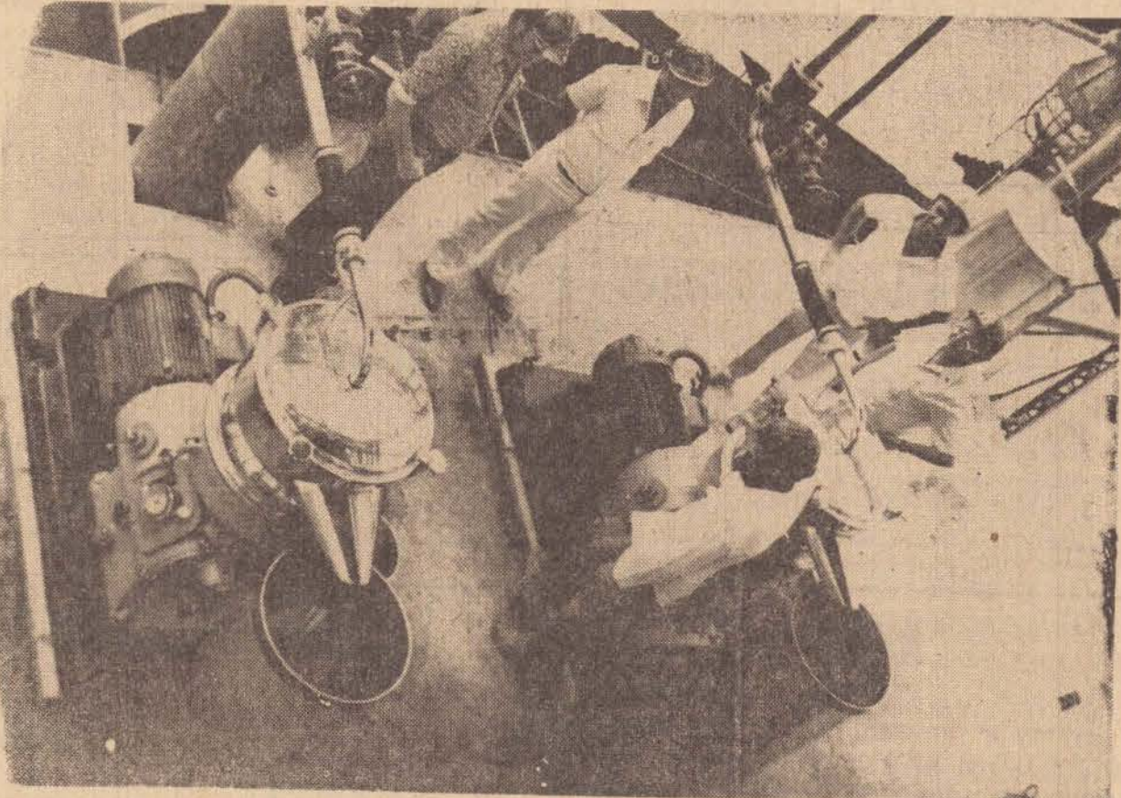
Num plano superior do prédio de destilação, nosso fotógrafo João Magalhães focalizou o setor das separadoras centrífugas. Essas separadoras tem como função, na Destilaria, a separação do fermento do caldo, após a fermentação das dornas. Ao centro, o engenheiro agrônomo José Fernandes, dando explicações sobre o assunto.
