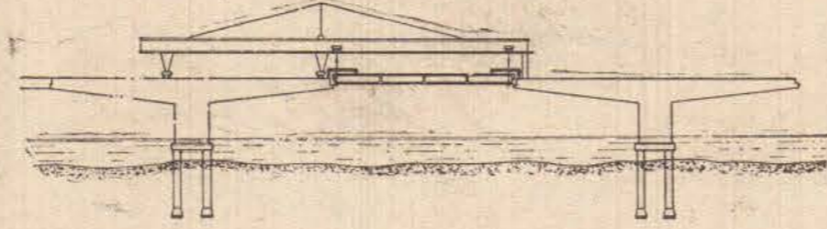
Modo de colocação das vigas premoldadas
