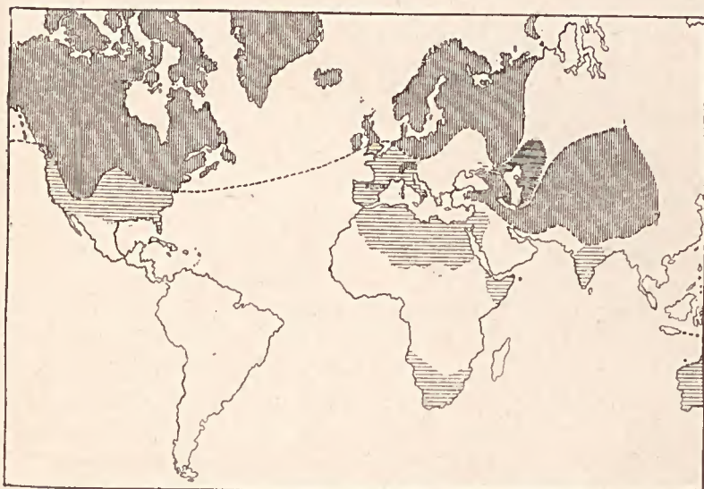
Fig. 136. — Les glaces et l'expansion de l'industrie paléolithique (Types chelléen et acheuléen).
