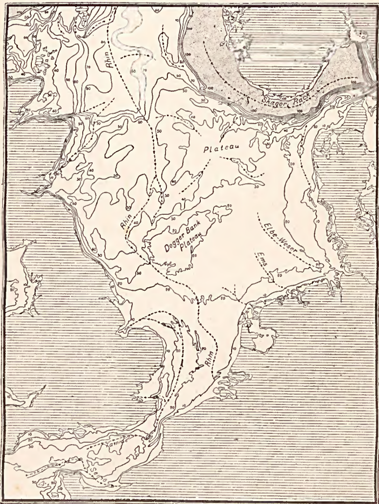
Fig. 3. — Le plateau sou-marin de la mer du Nord.
