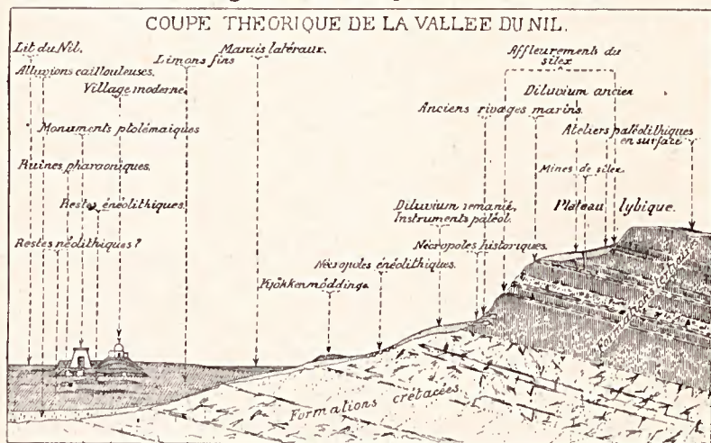
Fig. 1. — Coupe théorique de la vallée du Nil.
