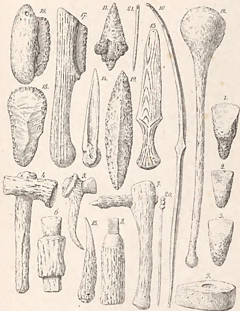
Fig. 31. — Outillage néolithique des Cités lacustres.
