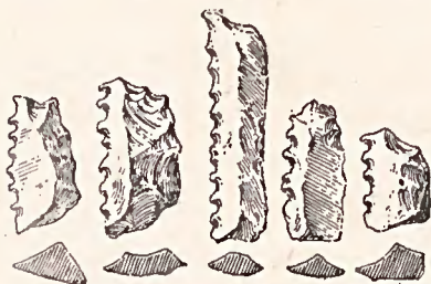
Fig. 92. — Abuchal, près Carmona (Espagne), d'après G. Bonsor.
