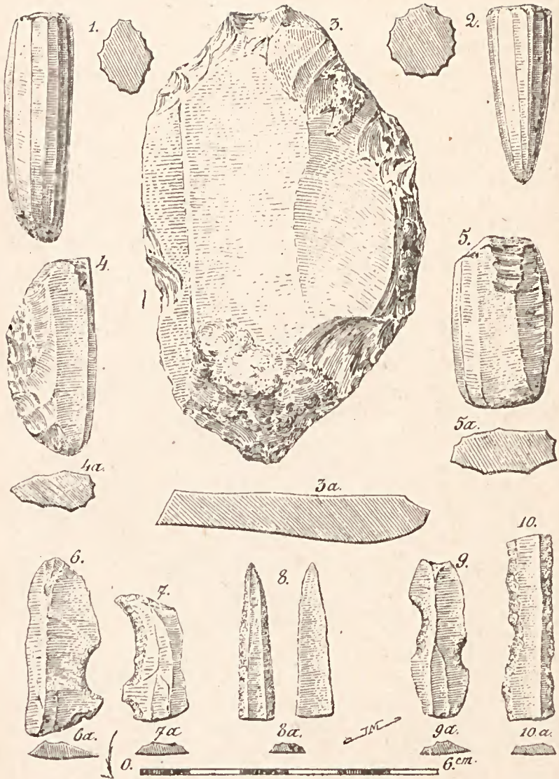
Fig. 49. — Tépeh Goulam (Poucht e Kouh).
