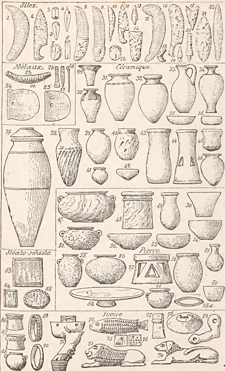
Fig. 48. — Industrie eneolithique des temps historiques en Egypte. Objets de la 1 re dynastie pharaonique.
