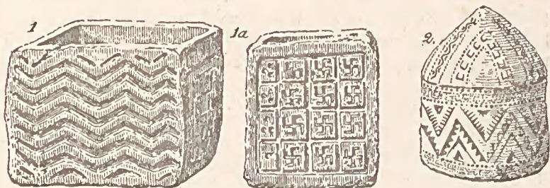
Fig. 132. — Poterie incisée. Nécropole de Djonu (Talyche russe).
