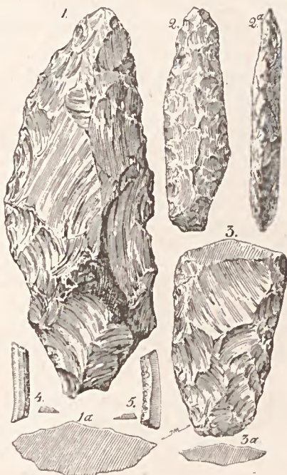
Fig. 38. — Instruments néolithiques, de la Palestine.
