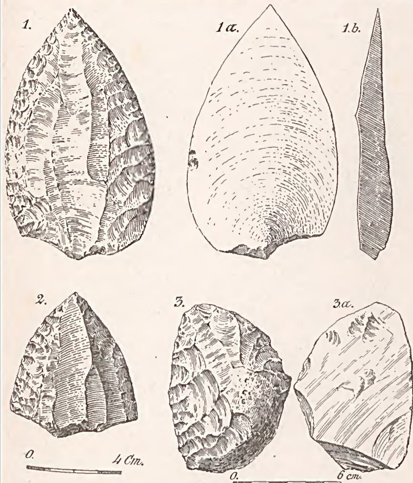
Fig. 15. — Instruments de type moustérien (Le Moustier).
