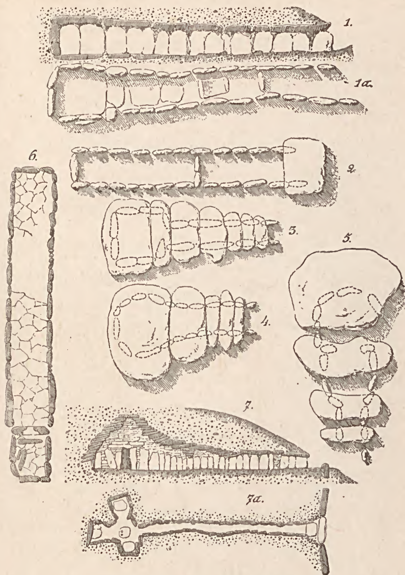
Fig. 146. — Dolmens, plans et coupes.
