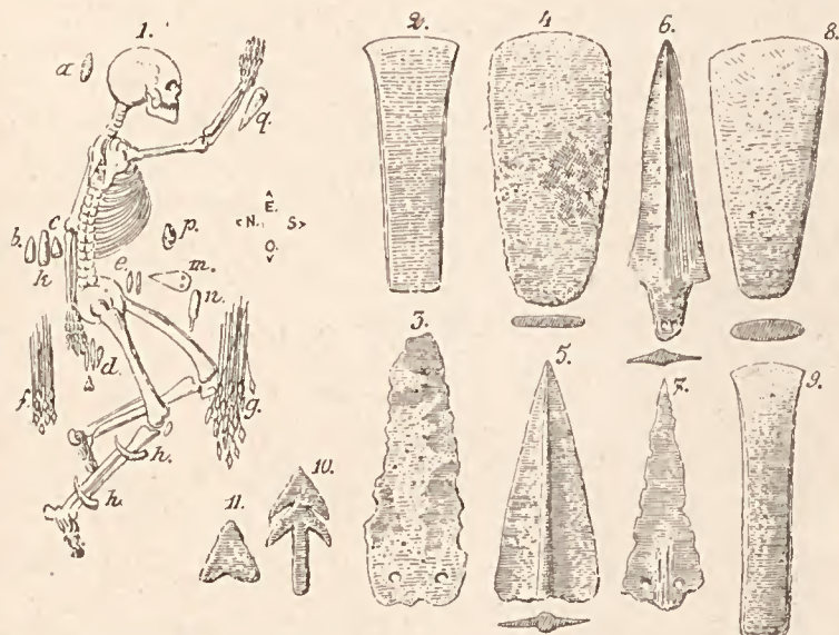
Fig. 50. — 1, Sépulture énéolithique de Fontaine-le-Puits (Savoie) — a, Pointe de javelot. — b, c, Haches en jadéite — d, Lames et tranchets. — e, Lames et grandes pointes de flèches. — f, 10 pointes de flèches en silex. — g, 22 pointes de flèches en silex — h, Défenses de sanglier. — k, Hache plate en cuivre (n° 2). — m, Poignard en cuivre (n° 3). — n, Poignçon en cuivre. — p, Coquillage. — q, Pendeloque en cuivre — 4, Suse, cuivre. — 5, Ile de Crète, id. — 6, Missarlik, id. — 7, Espagne (cuivre). — 8-11, Adimeiyeh (Égypte), id.
