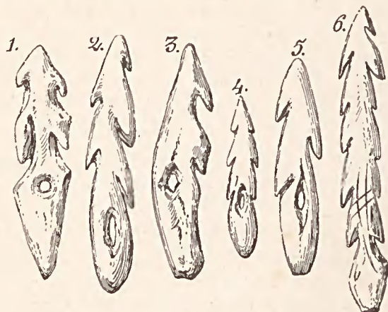
Fig. 26. — Harpons en os et en bois de cerf. — 1-3, Mas d'Azil. — 2-4, Grotte de la Tourasse (H e -Garonne) — 5-6, Grotte de Reilhac (Lot).
