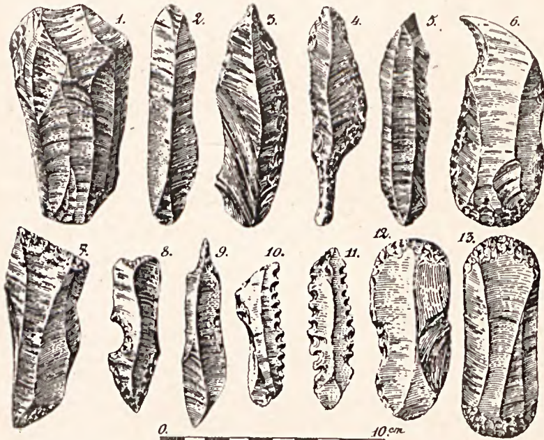
Fig. 22. — Industrie magdalénienne (types principaux de silex taillés).
