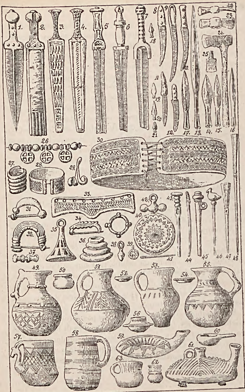
Fig. 66. — Industrie du fer, Arménie russe.
