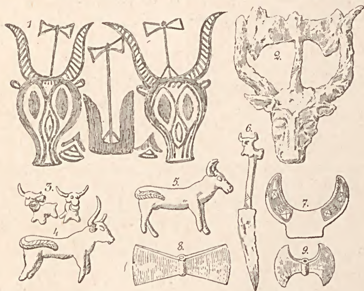
Fig. 162. — Haches et taureaux votifs : 1, vase mycénien de Chypre; 2, Ilissarlik; 3, Bythin (province de Posen); 4, 5, Chatillon-sur-Seiche (Ille-et-Vilaine); 6, Ilissarlik; 7, Ebersberg; 8, Olympie; 9, Grotte de Dicté (Crète).
