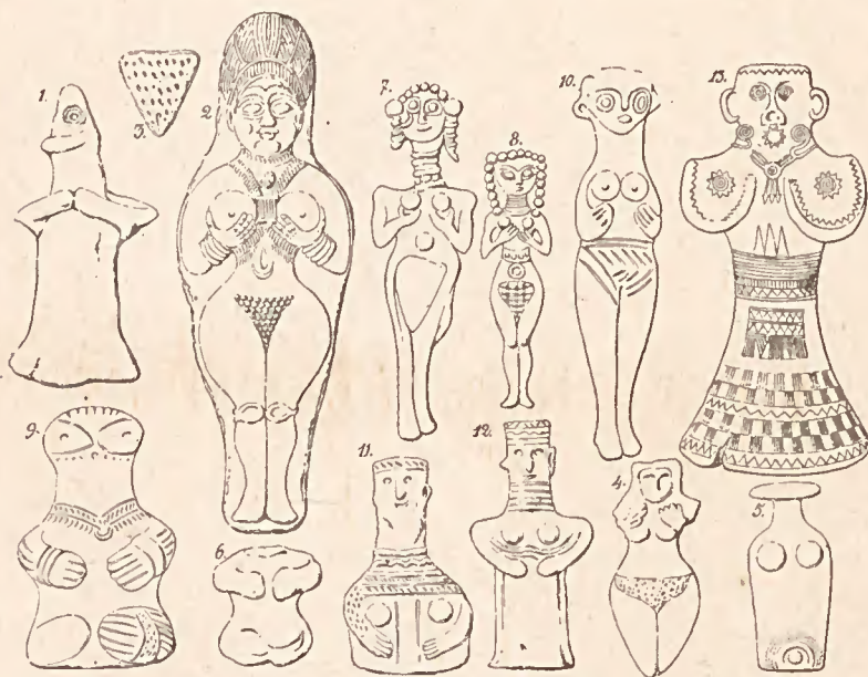
Fig. 156. — Représentations de la déesse Nana (Astarté).
