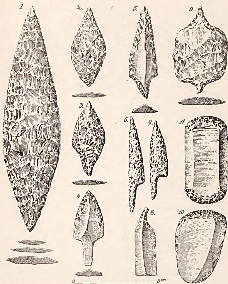
Fig. 21. — Industrie solutréenne. Types principaux de silex taillés.
