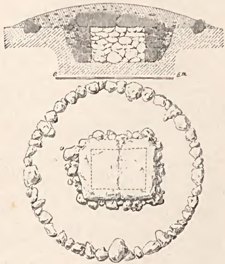
Fig. 148. — Dolmen bâti de Námia, province d'Ardébil (Perse) [relevés de l'auteur].
