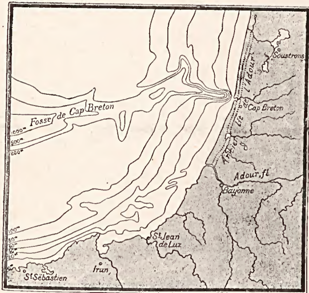
Fig. 2. — La fosse de Cap Breton.
