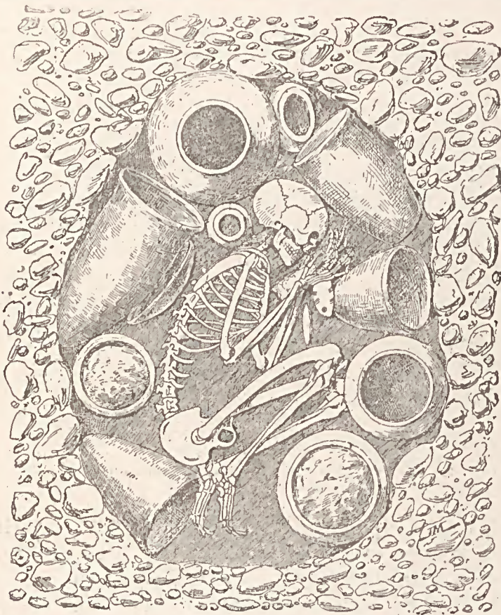
Fig. 141. — Sépulture néolithique d'El-Amrah (Haute-Égypte).
