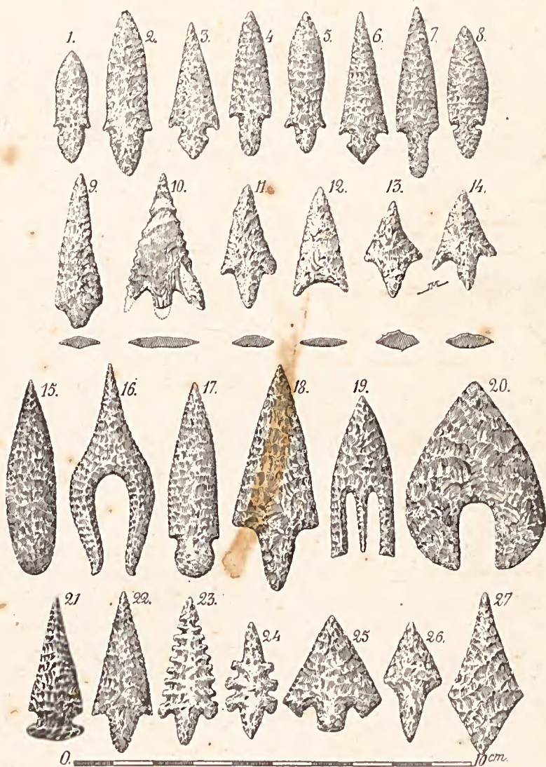
Fig. 28. — Pointes de flèches. — 1-8, Abydos (Coll. de Pateur, don au Musée de St-Germain). — 9-14, Ouargla (récolte Pézard). — 15, Suse (Musée de St-Germain). — 16, Alcala (Portugal) — 17, Gironde (S.-G.). — 18, Aveyron (S.-G.). — 19, Dolmen de Gourillach (Finistère) — 20, Fayoum. — 21, Californie (obsidienne). — 22, Aveyron. — 23, P (id). — 24, Finistère. — 25, Loir-et-Cher. — 26, Abruzzes (Italie). — 27, Aube.
