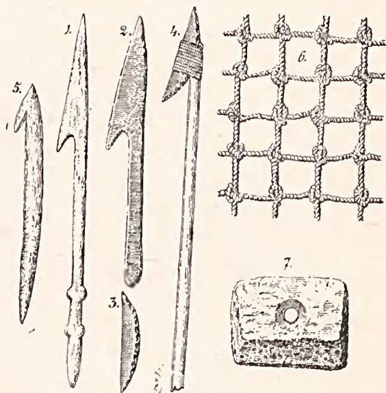
Fig. 83. — Harpons et instruments de pêche. — N° 1, Ivoire. N° 2, Cuivre (Abydos). N° 3, Silex (Hélouan). N° 4, Emmanchement du n° 3. N° 5, Corne de cerf (Iac de Neuchâtel). N° 6, Robenhausen (Suisse). N° 7, Flotteur en bois de pin (Robenhausen, Suisse). (N°s 5, 6, 7, d'après A. de Mortillet.)
