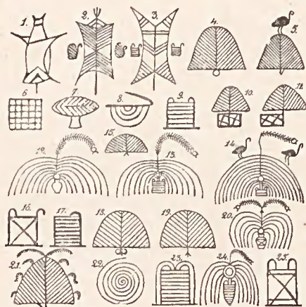
Fig. 151. — Emblèmes religieux et insignes des tribus sur les vases peints prédynastiques d'Égypte. 1 à 13, Negadah et Ballas ; 14, El-Amrah et Abydos ; (15 à 21, d'après Schweinturth).
