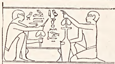
Fig. 77. — Bas-relief de la VI e dynastie d'Égypte. La fabrication des vases de pierre.
