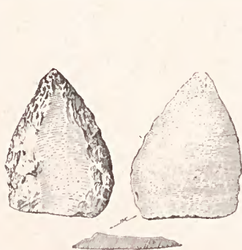
Fig. 16. — Pointe de type moustérien. Silex blond. Oasis de Kharghiyeh (Égypte).
