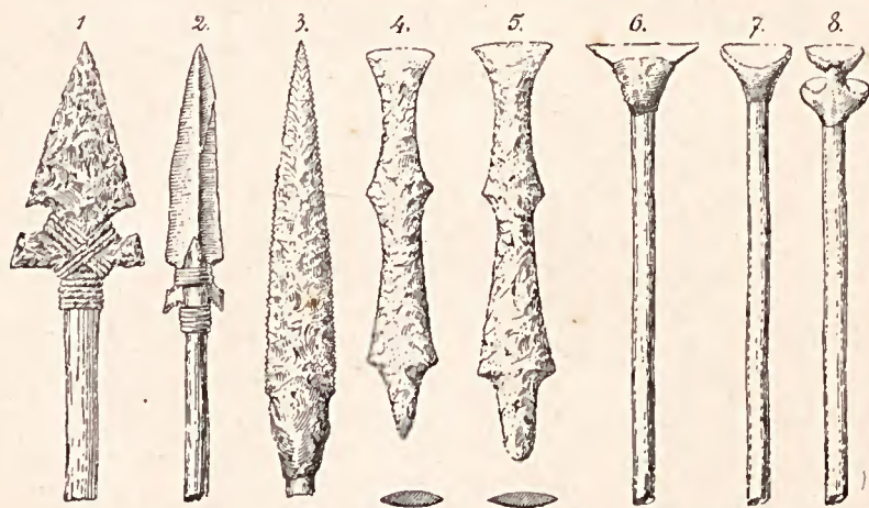
Fig. 41. — Emmanchement des pointes de flèches en silex.
