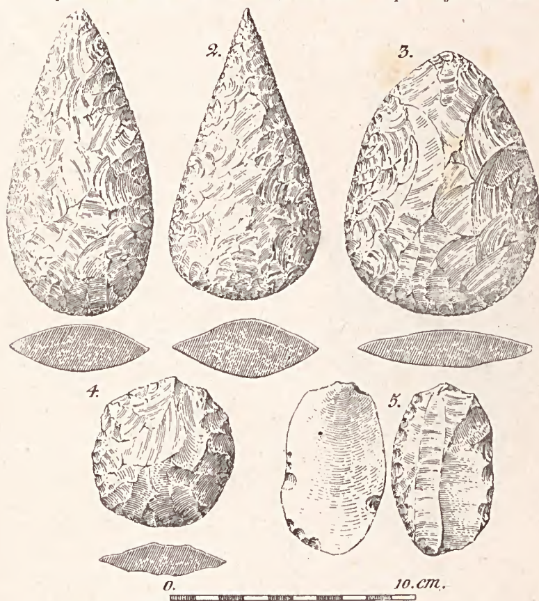
Fig. 9. — Instruments de type acheuléen (S t -Acheul).
