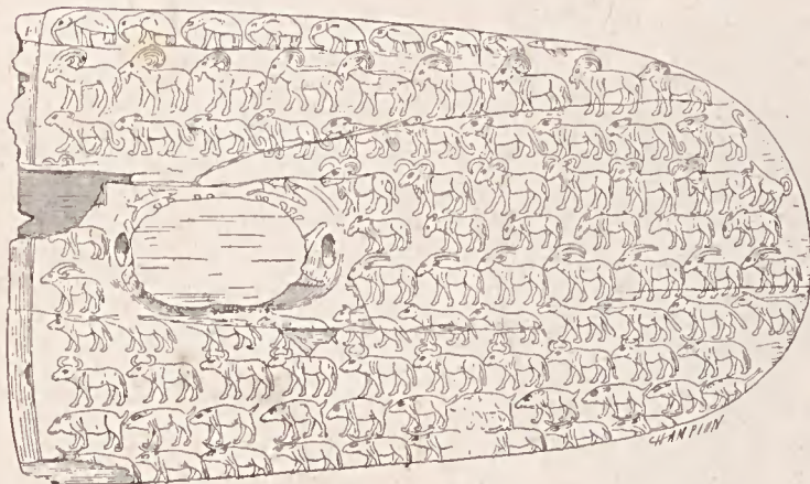
Fig. 121. — Manche en ivoire de poignard en silex, représentant la faune de l'Égypte au temps du début du régime pharaonique (découverte de Henri de Morgan à Ilassaya, près d'Edfou). Lignes à partir du haut. 1. Éléphants; 2, Autruches, Girafes; 3, Panthères; 4, Capridés; 5, Chacals; 6, Antilopes; 7, Porcs-épics; 8, Bœufs; 9, Hippopotames; 10, Antilopes; 11, Éléphants, Salmonidés; 12, Capridés; 13, Panthères; 14, Capridés, Chien; 15, Anes; 16, Antilopes; 17, Chiens et Chacals; 18, Bœufs; 19, Porcs ou Sangliers; 20, Bœufs.
