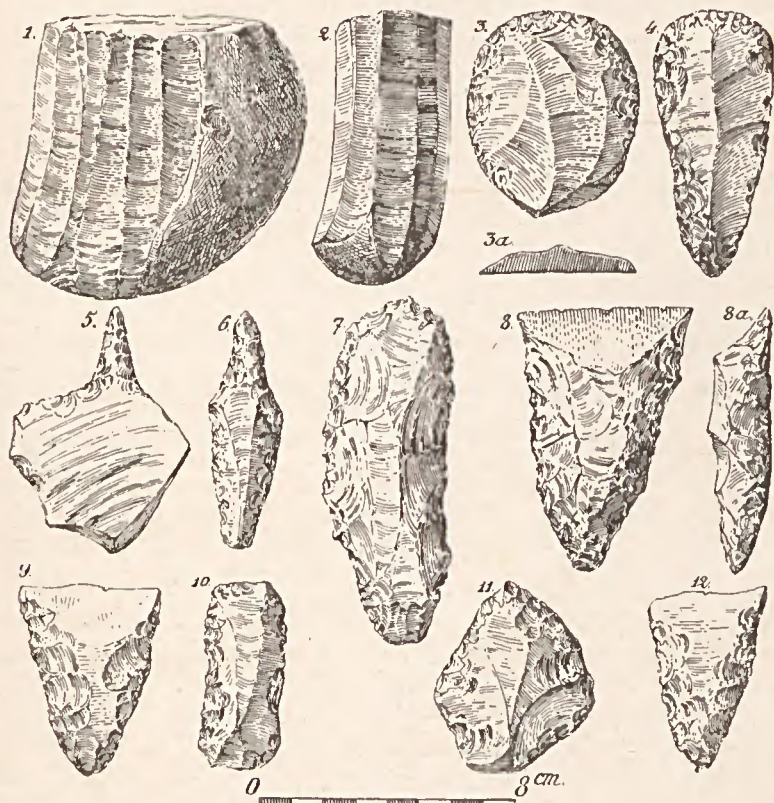
Fig. 27. — Silex taillés campigniens (Le Campigny, Seine-Inférieure).
