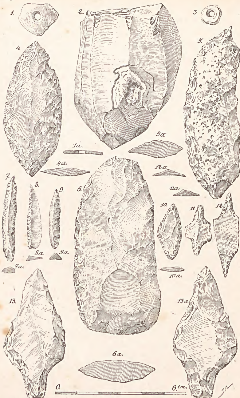
Fig. 37. — Néolithique du Sahara (Rech. Pézard) (environs de Ouargla). — 1 et 3, Coquille d'œuf d'autruche. — 2, Silex blond opaque. — 4, Silex brun.
