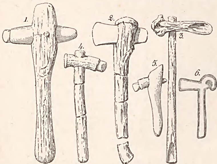
Fig. 40. — Emmanchement des haches de pierre polie.
