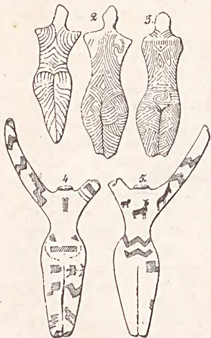
Fig. 96. — 1 à 3, Figurines d'argile, dessins gravés (Iassy, Roumanie). — 4 à 5, Figurines d'argile, dessins peints (Toukh, II e -Égypte).
