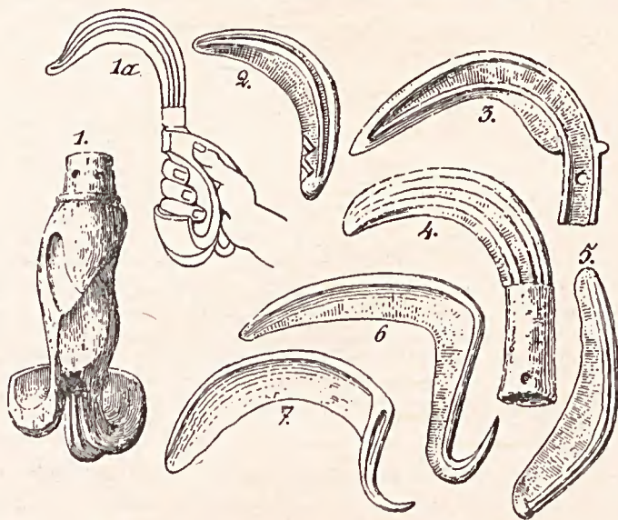
Fig. 93. — Faucilles de bronze : 1, Palafitte de Moringen (Suisse) ; 2, Corcelette ; 3, Guévaux ; 4, Athlone (Wessmeath) ; 5, Jura ; 6, Hongrie ; 7, Caucase.
