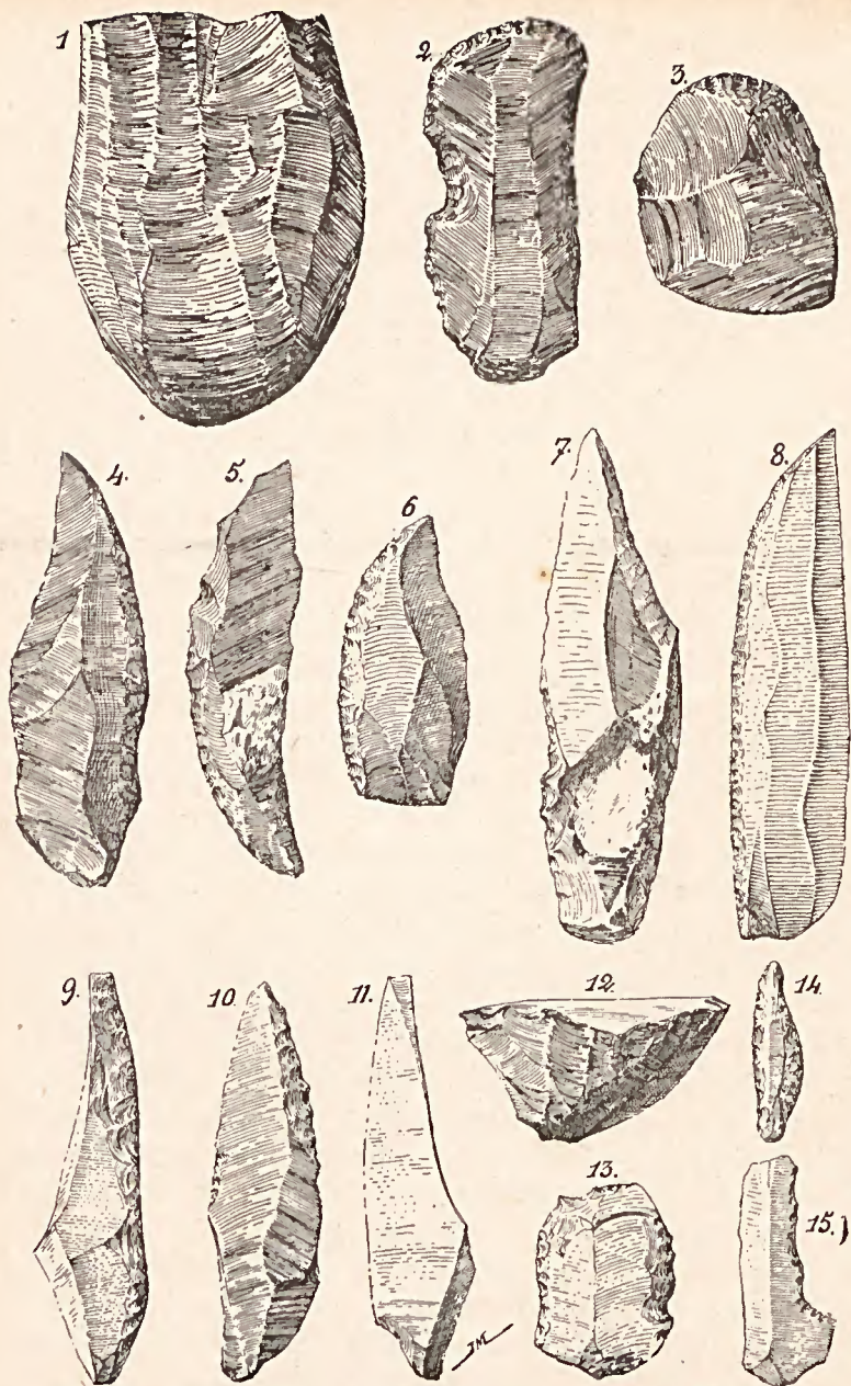
Fig. 24. — Silex taillés de l'industrie capsienne. — 1 à 8, El Mekta (Tunisie). — 9 à 15, Foun el Maza (Tunisie).
