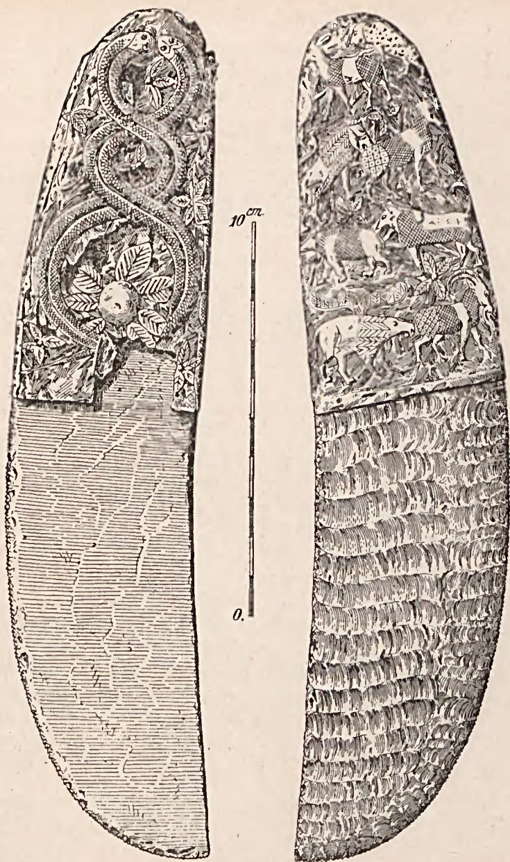
Fig. 125. — Couteau de silex blond garni d'une feuille d'or ornée au repoussé Nécropole de Saghel-el-Baglieh (?), Haute-Egypte (Musée du Caire).
