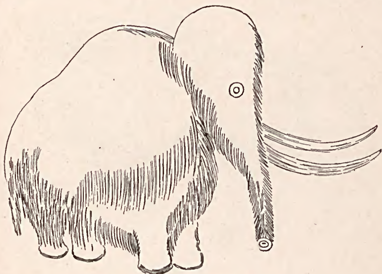
Fig. 102. — Mammouth (Font de Gaume).
