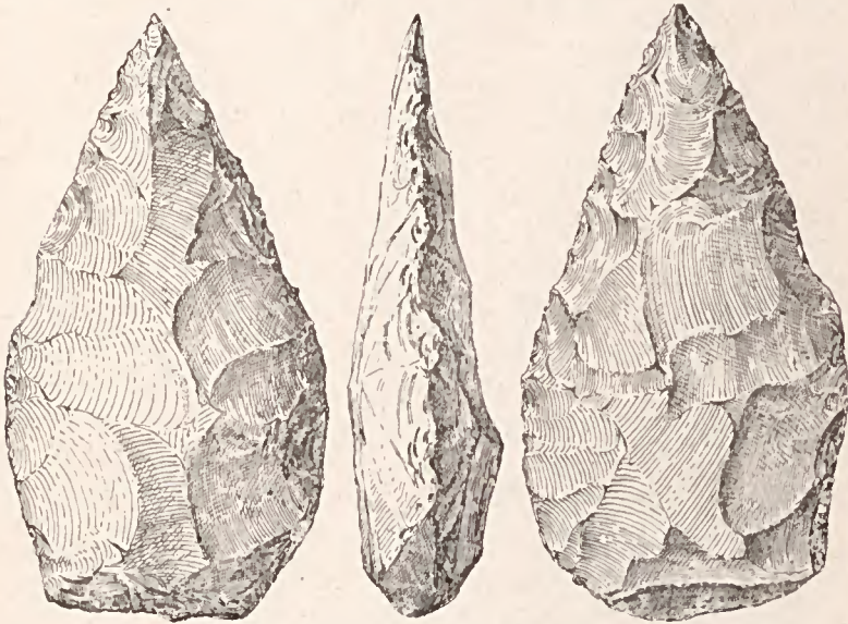
Fig. 11. — Instruments de type acheuléen (Tunisie).
