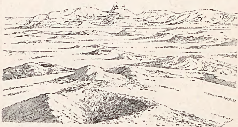
Fig. 74. — Mines de silex de Ouadi el Cheikh, d'après une photographie de H.-W. Seton Karr.
