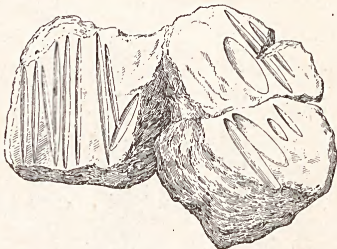
Fig. 76. — La « Pierre aux dix doigts », Villemaure (Aube).
