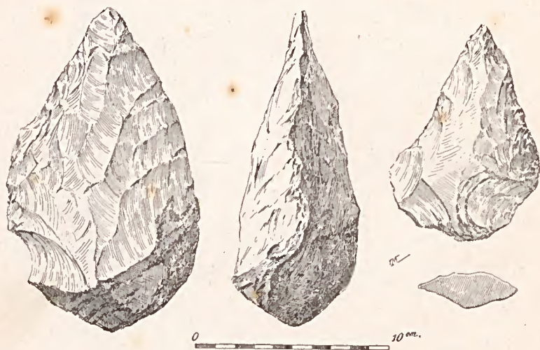
Fig. 13. — Instruments de type chelléen et acheuléen (Somal).
