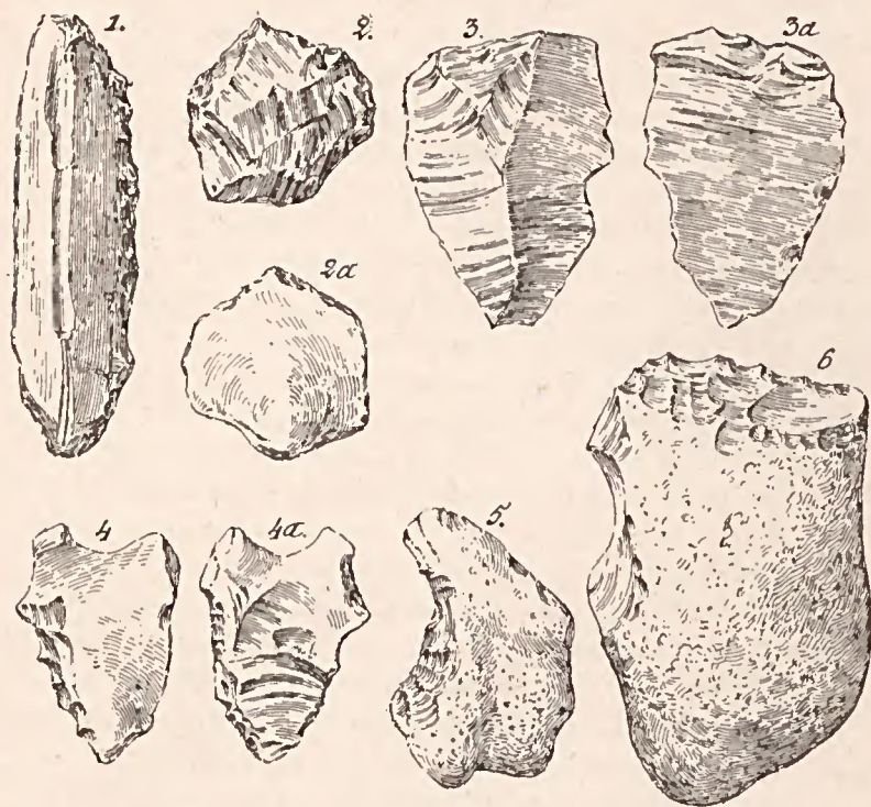
Fig. 7. — Eolilhes . 1, 2 et 2a, Thenay (Loir-et-Cher). — 3 et 3a, Otta (Portugal) — 4 et 4a, Puy-Courny. — 5 et 6, Belgique.
