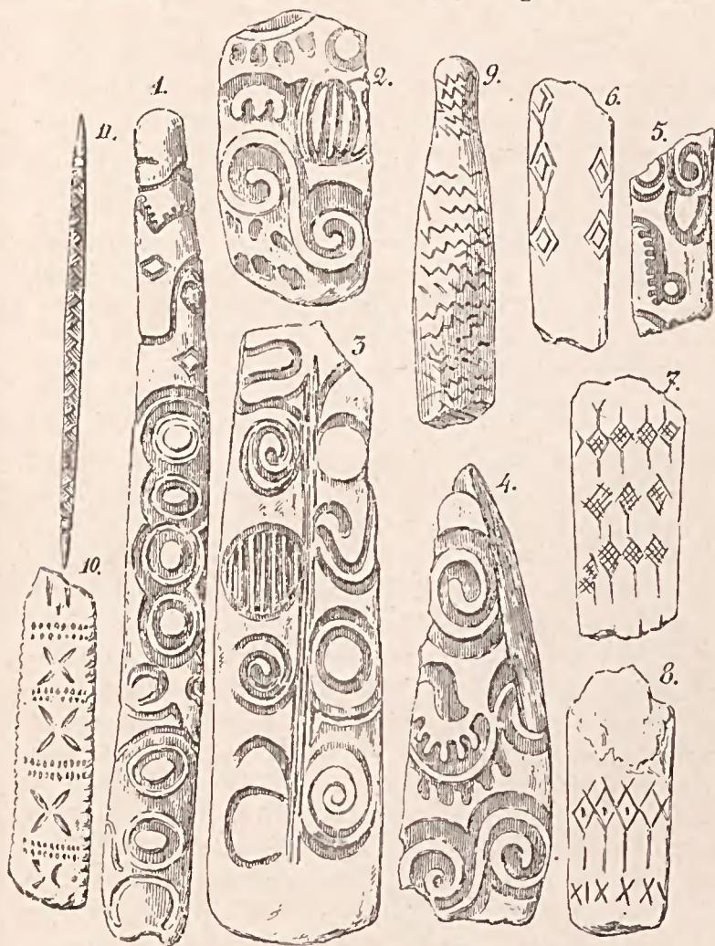
Fig. 116. — Dessins magdaléniens de type géométrique.
