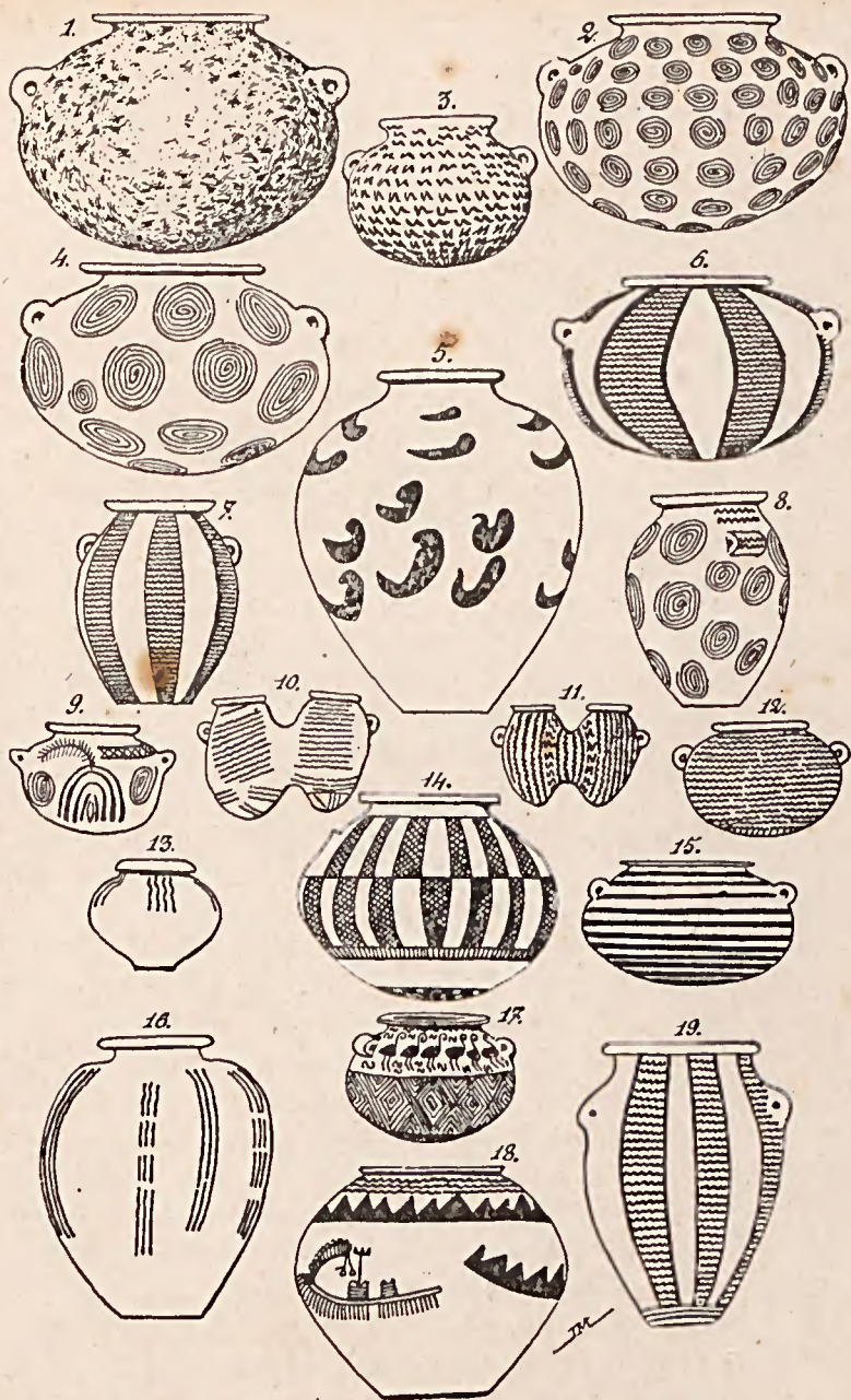
Fig. 122. — Céramique égyptienne pré-dynastique.
