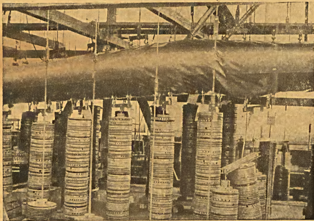
Cuidadosos ensaios de carga em peças de aviões. A fotografia mostra uma seção de ensaio especial das fábricas de aviões Dornier, em que se fazem experiências de resistência de uma asa de aeroplano, carregando-a de chapas de aço de que cada uma pesa 10 quilos.
