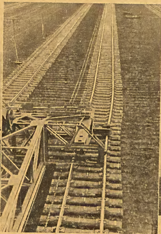
E' esta a instalação reversora da ponte de terraplanagem a qual assenta, automaticamente, de cada vez, a via permanente.
