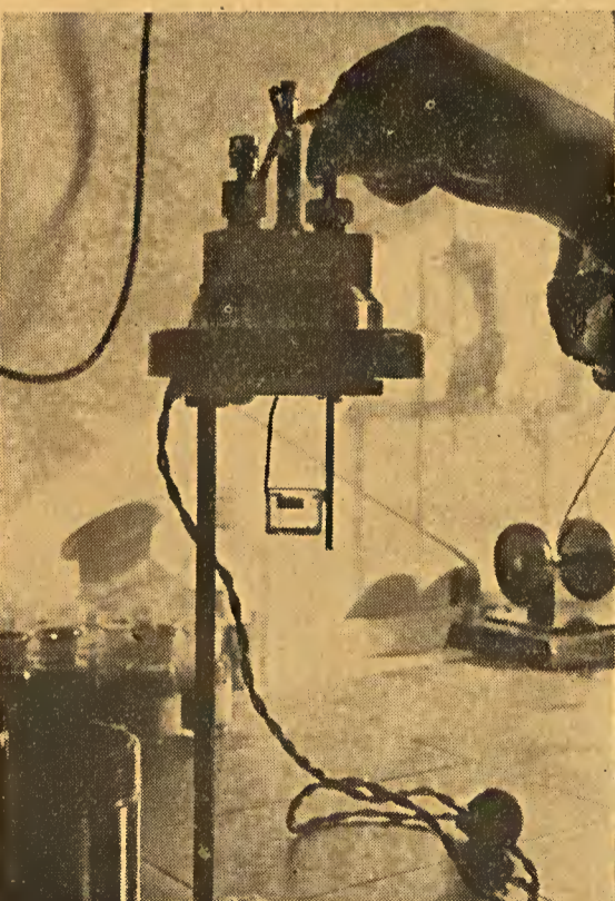
Para a determinação do valor calorífico, faz-se a combustão elétrica de uma partícula de lignito dentro de uma bomba de oxigênio e mede-se a temperatura originada.
