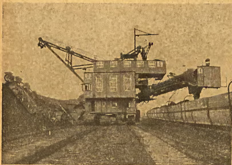
Uma draga de rosário em funcionamento numa mina de lignito. A' direita cai o lignito carregado pela correia transportadora para dentro de grandes vagonetes.
