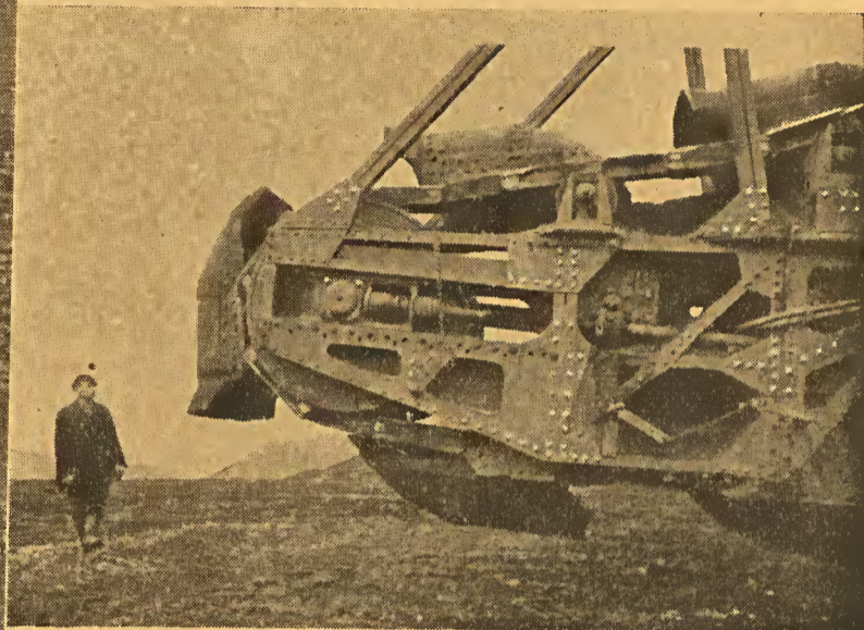
O rosário da ponte de terraplanagem ao dragar a espessa camada de areia que encobre o lignito.
