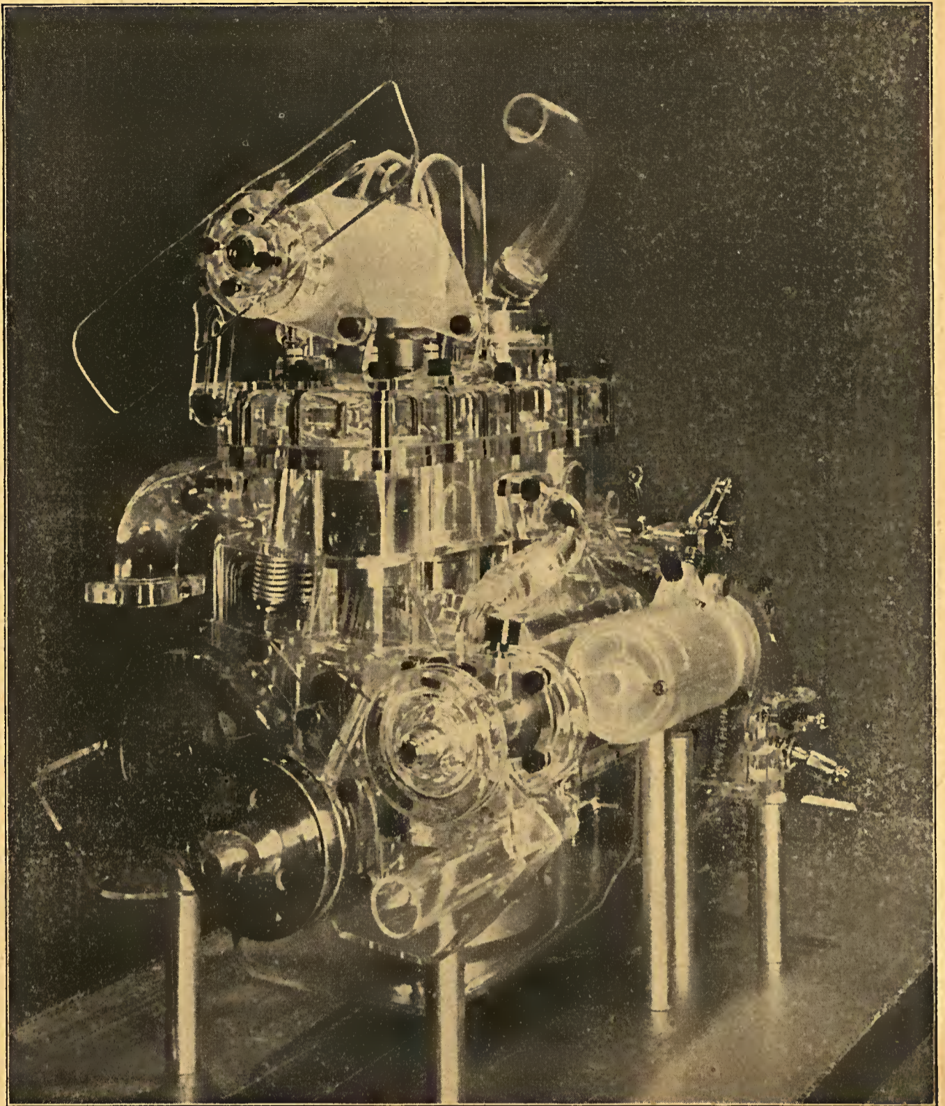
Os segredos do processo de funcionamento de máquinas são revelados em motores, relógios, máquinas de escrever, aparelhos de medição etc. construídos de plexi. Mostra a gravura o aspecto que oferece um motor construído com vidro plexi alemão.
