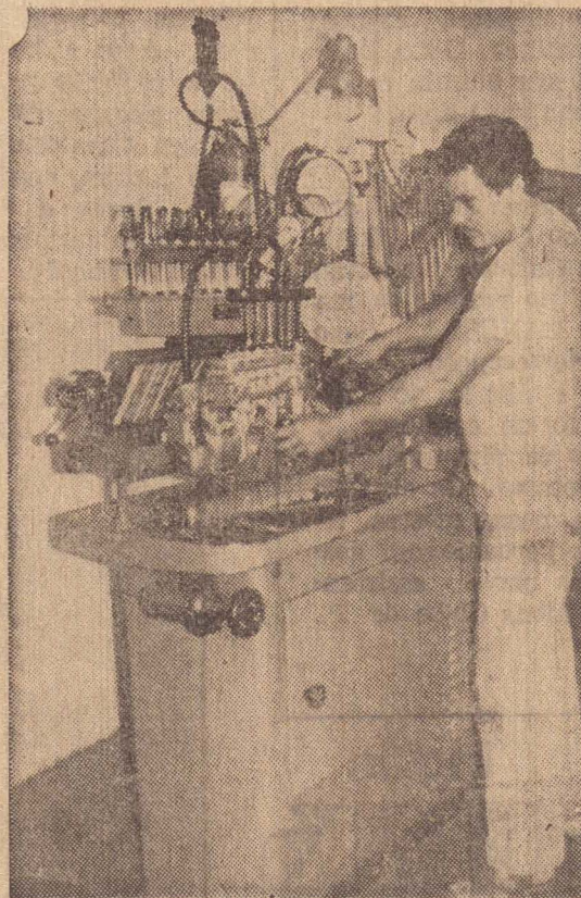
Aparelho de testes de bombas injetoras de Silva é o operador e salientou a importância fabricação alemã "Bosch". José Carlos da deste aparelho que é importante para o controle de economia de combustível e o bom funcionamento do motor, garantindo maior potência
