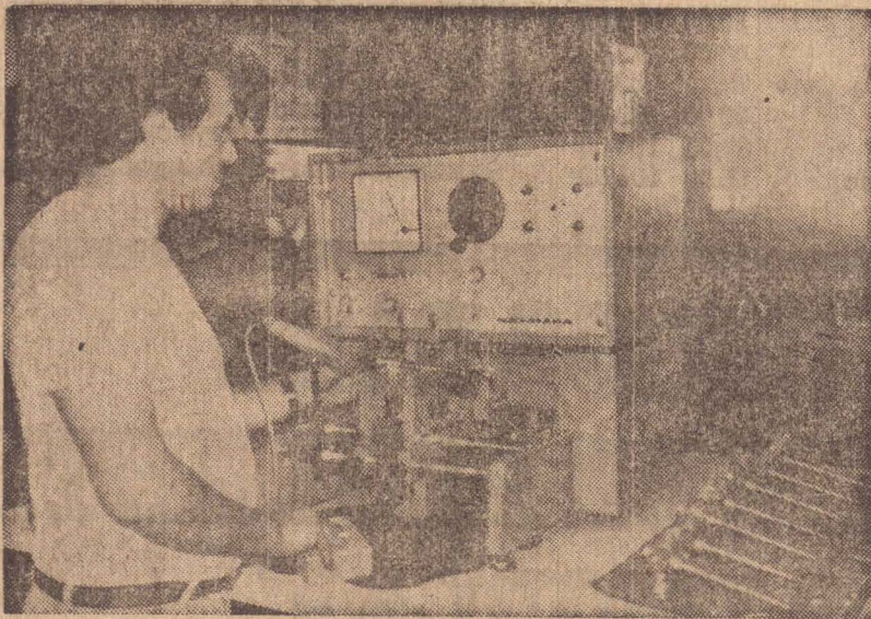
Máquina eletrônica HOFMANN para balanceamento de eixos de turbinas. Única no interior e que garante maior aproveitamento dos motores garantindo 10% de economia de combustível. Seu operador é Geraldo Sacramento
