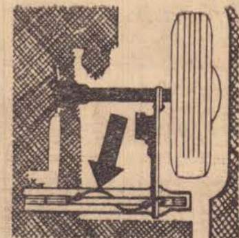
Suspensão por barras de torção, independente nas 4 rodas - a mais macia e mais resistente.
