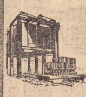
FÔRNO ELÉTRICO G&M DE MALEABILIZAÇÃO
