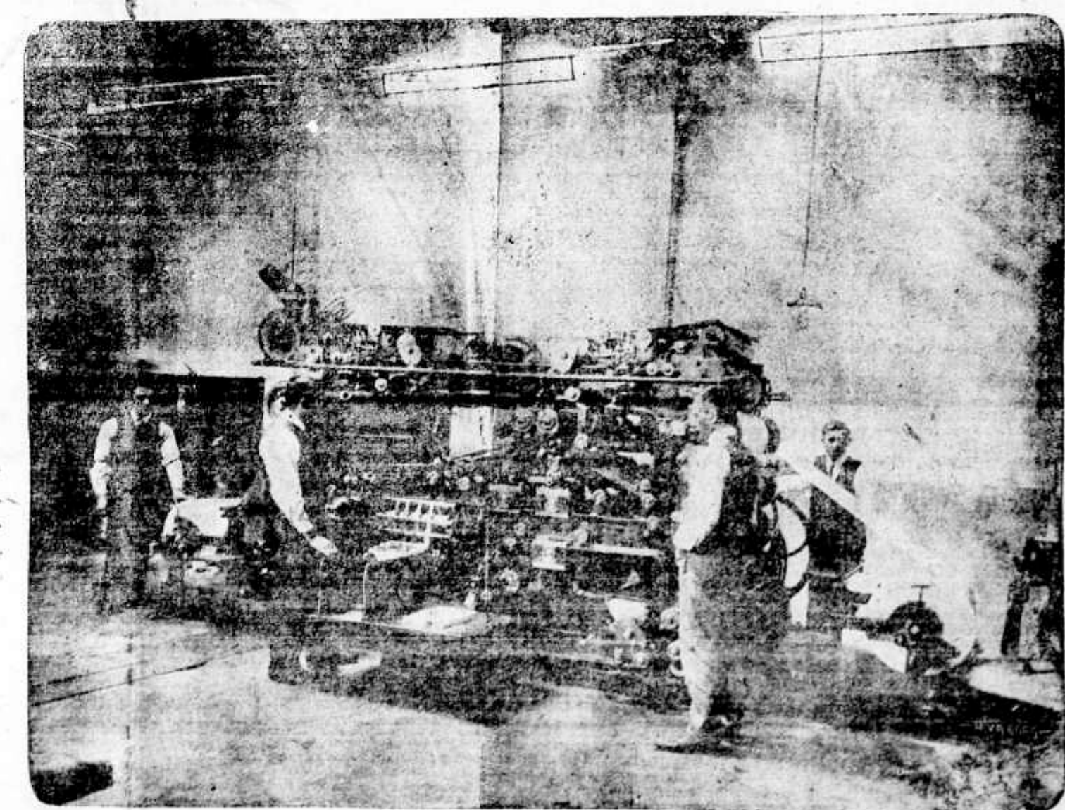
MACHINA ROTATIVA DE MARINONI, ONDE É IMPRESSO O «COMMERCIO DE SÃO PAULO»
