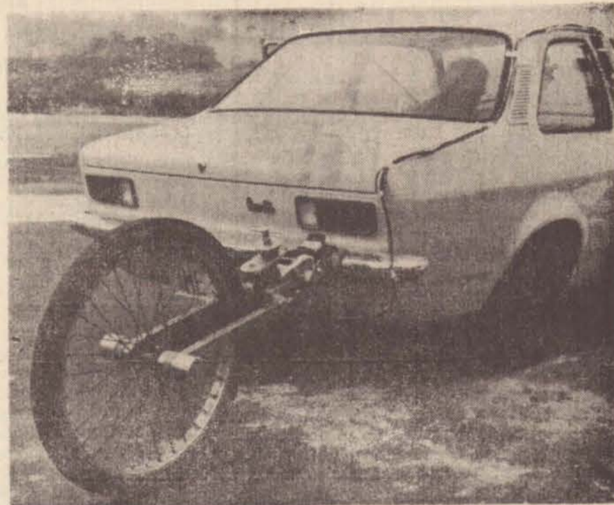
A quinta roda determina, com precisão, a velocidade e distância de parada do veículo.
