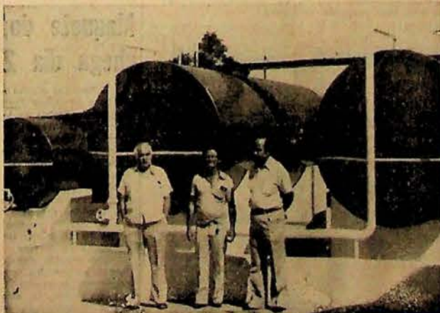
Um conjunto de tres tanques, os dois primeiros quinze mil litros e terceiro 5 mil litros para óleo diesel. São vistos Mauro Gomes, Antonio Almodova e Silvio Pullig.
