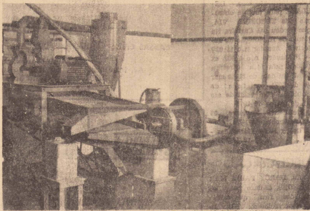
O mais moderno maquinário foi adquirido pelos Irmãos Rodrigues para as Máquinas Andrés Ltda., que esta semana deverá passar a produzir os mais diversos artigos de feccularia.
