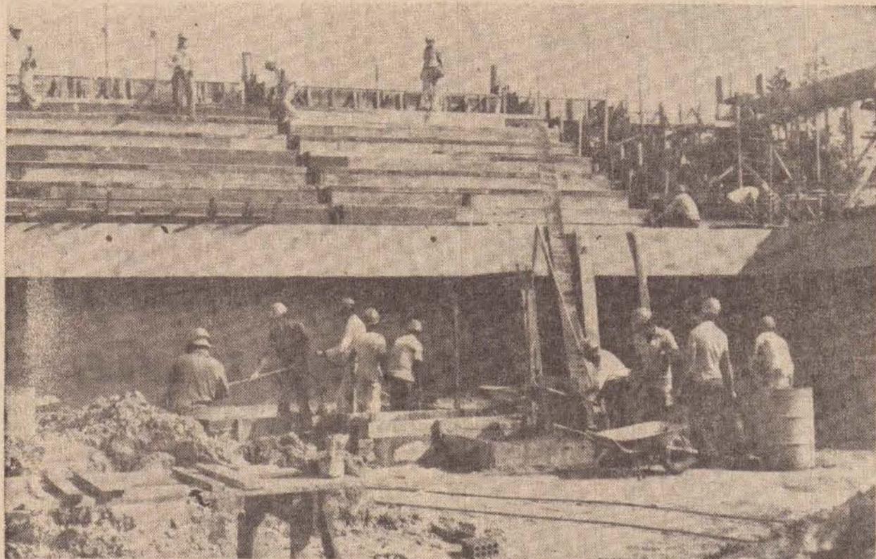
Aspecto da preparação para concretagem do 1.º lance de arquibancada do Ginásio de Esportes da APEC.
