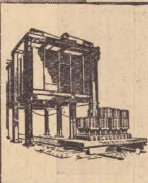
FÔRNO ELÉTRICO G&amp;E DE MALLEABILIZAÇÃO
